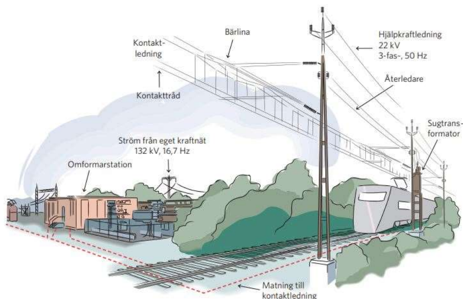
Figur 5.1-1. Järnvägens elanläggning.
