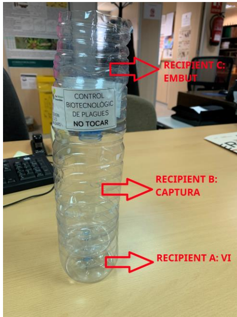
Fig. 13. Trampa muntada. Fig. 13. Mounted trap.
