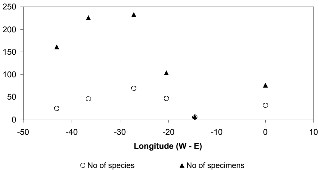
Fig. 9.18: Longitudinal trends
