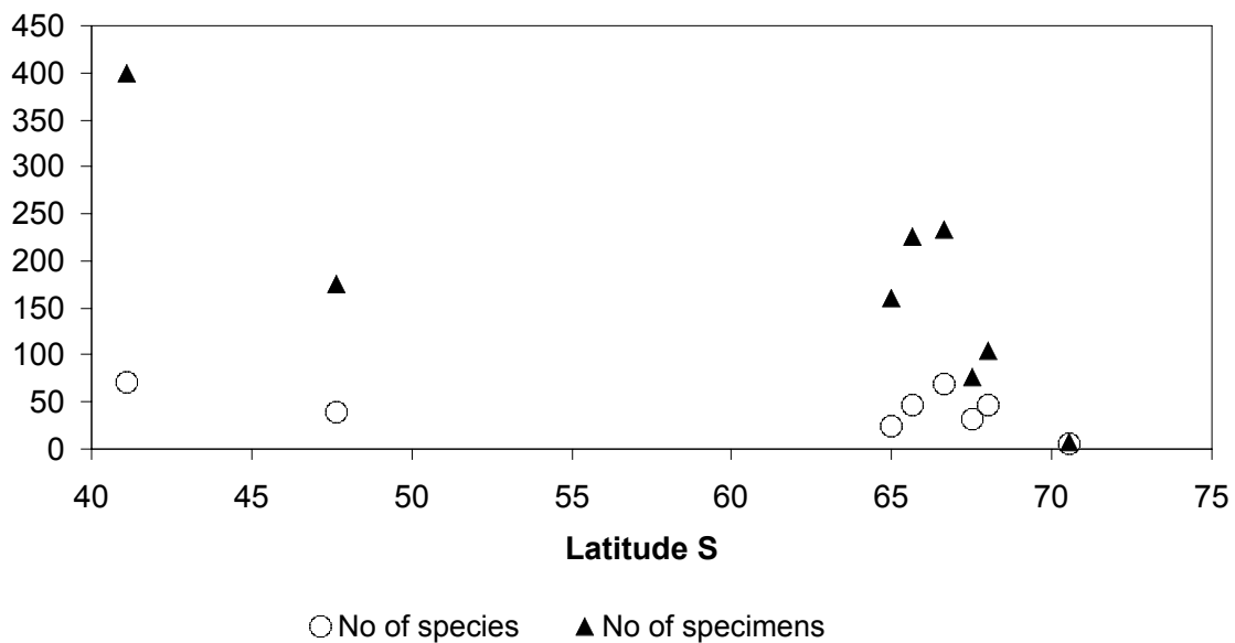
Fig. 9.17: Latitudinal trends
