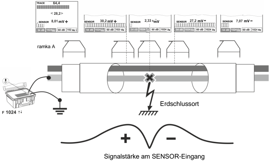
Abb. 38. Anschlussschema und Signalstärke für die Methode der Isolationschadenverfolgung mit Isolationskontrolle
