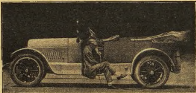
Nuevo sistema de hinchar los neumáticos automáticamente
