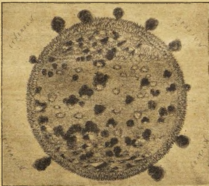
Esquema del Sol, tal como fué observado en Roma, en 1635, por Scheiner
