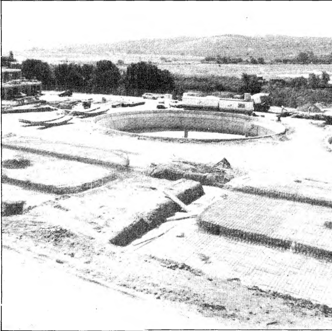
La nueva planta depuradora cuenta con varios decantadores de once y quince metros de radio y 3,5 de alto.
