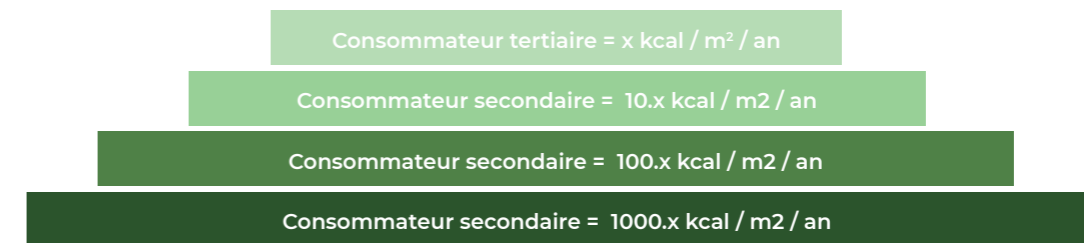
Figure 4 : Illustration du principe de construction de bas en haut à travers l'exemple des pyramides trophiques et de la loi de Lindemann
