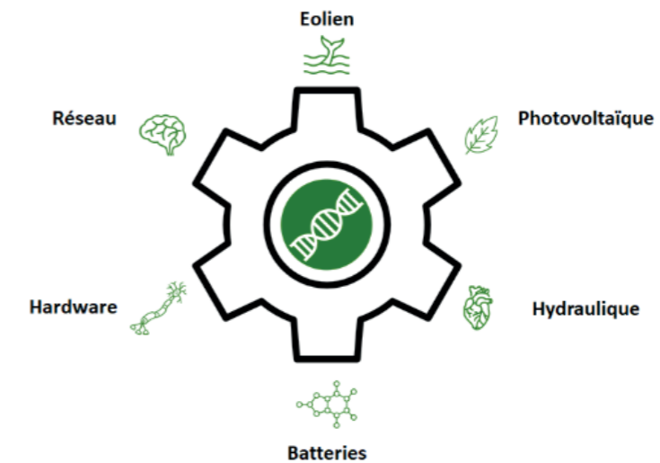
Figure 2. Illustration des convergences entre les besoins fonctionnels technologiques et biologiques © Ceebios
