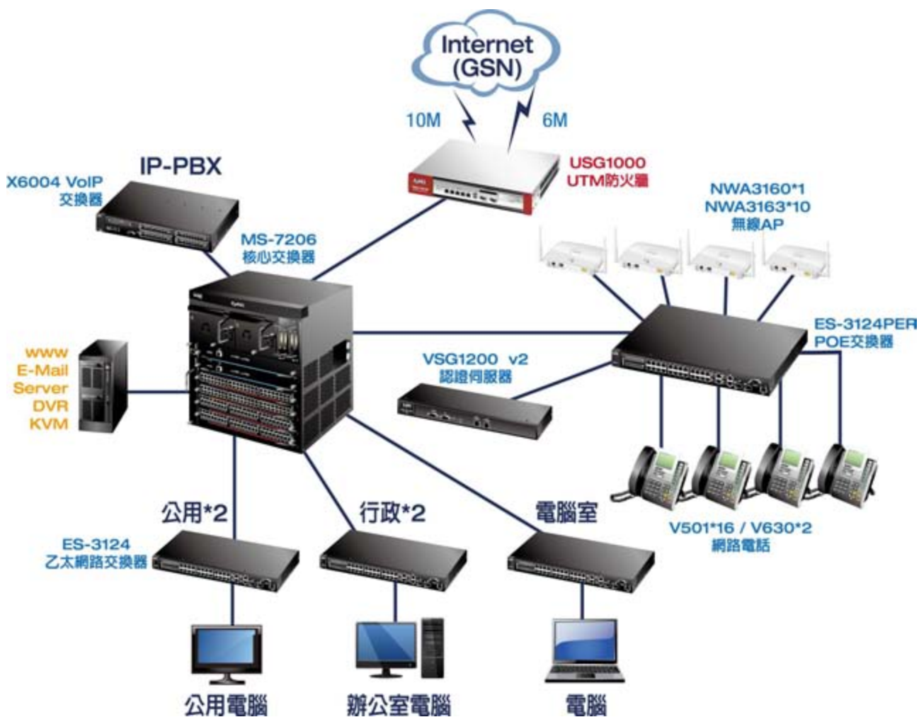
圖 / 台中縣圖書資訊中心網路架構
