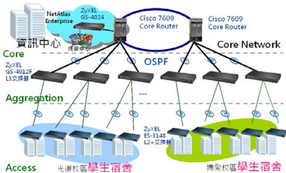
圖 / 交通大學宿舍網路架構
