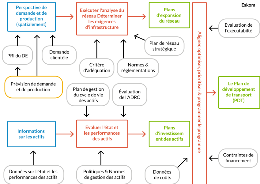
Figure 9.4 : Processus de planification du développement du réseau de transport d'Eskom
