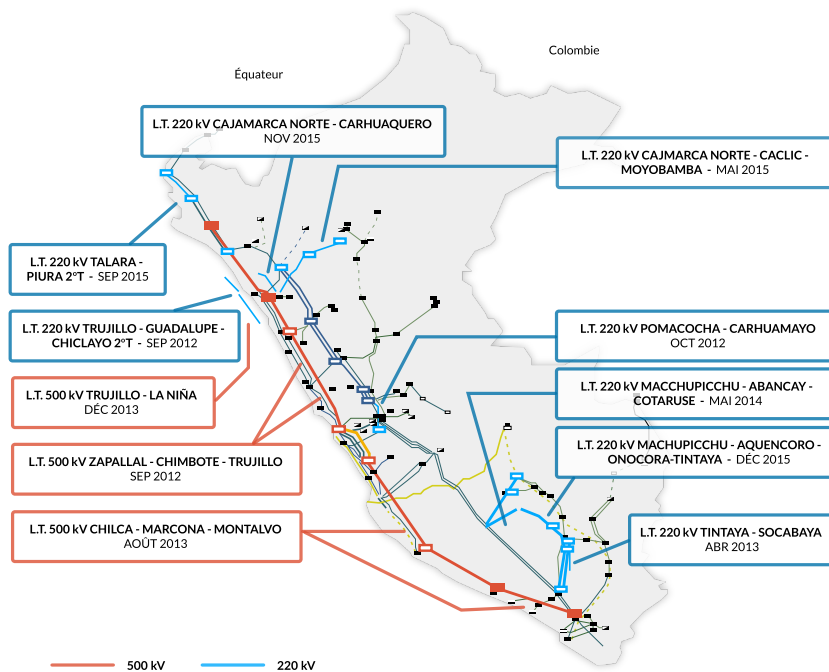
Figure 5.2 : Lignes de transport au Pérou (Source : Pedro E. Sanchez, Banque mondiale 2018)
