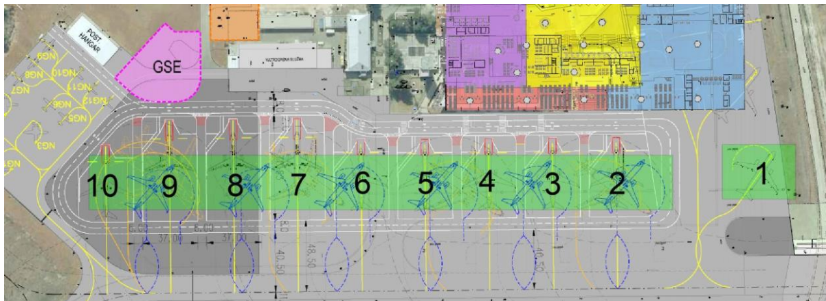
Slika 2. Predloženi jednoredni sustav parkiranja zrakoplova
