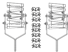
RUEDA ESCARDADORA DOBLE
