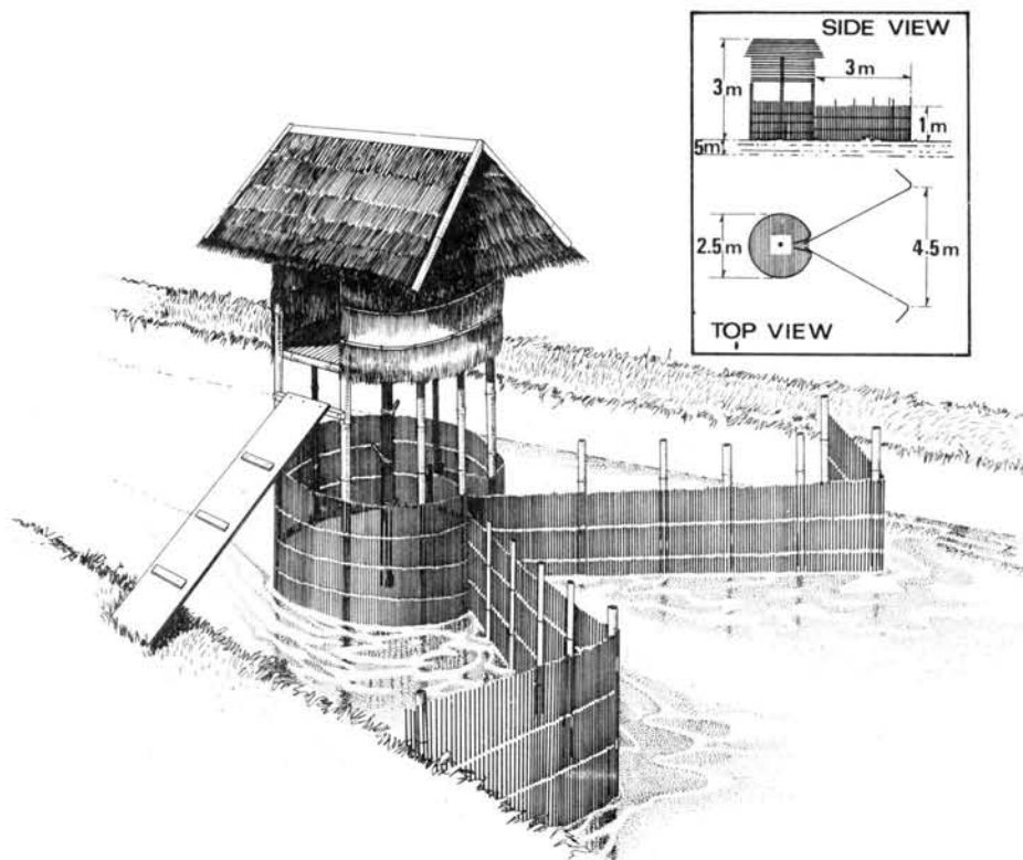
Fig. 19. Prawn trap.
