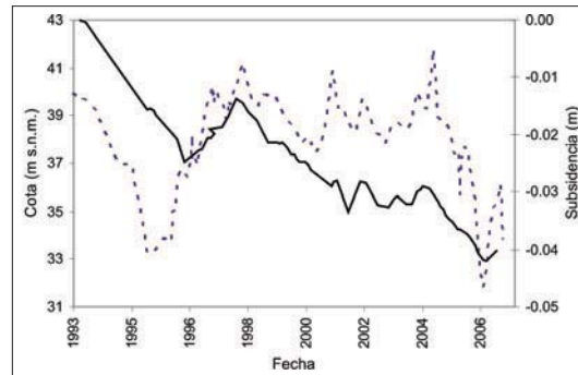
Fig. 18. Evolución temporal de la subsidencia (continua) y del nivel piezométrico (puntos) en un pozo situado al SW de la ciudad.
