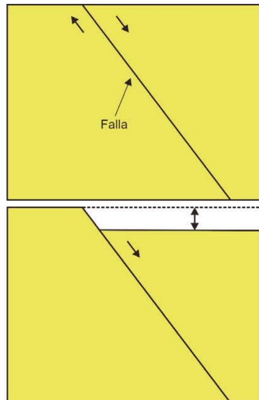
Fig. 9. Subsidencia tectónica.
