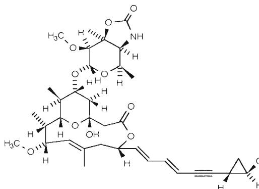
194 : Callipeltoside A
