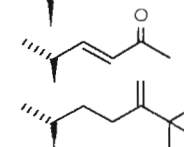
314 : R =
