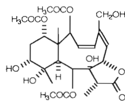
161: Labouteine
