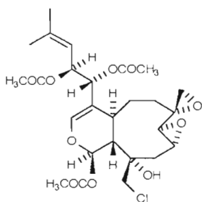
131 : Havannahine
