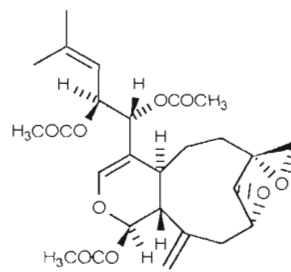
132, 133, 134 : Desoxyhavannahine
