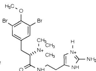
182 : B
