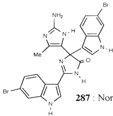
284 : Agelastatine A
