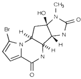
284 : Agelastatine A
