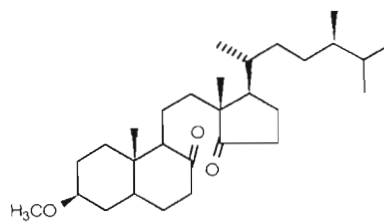
319 : Jereisterol B
