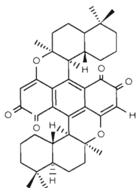
211 : Dipuupehedione
