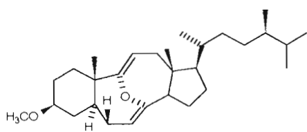
318 : Jereisterol A
