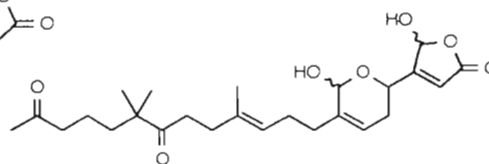
207 : Faciospongide B
