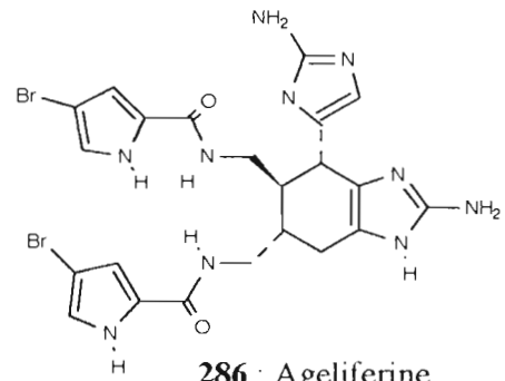
286 : Ageliférine
