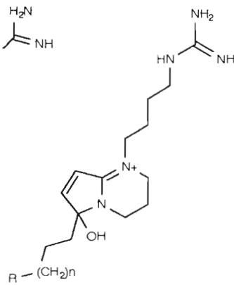
300 : Phloeodictine C1
