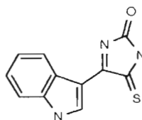
308 : Zyzine
