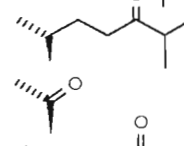
312 : R =
