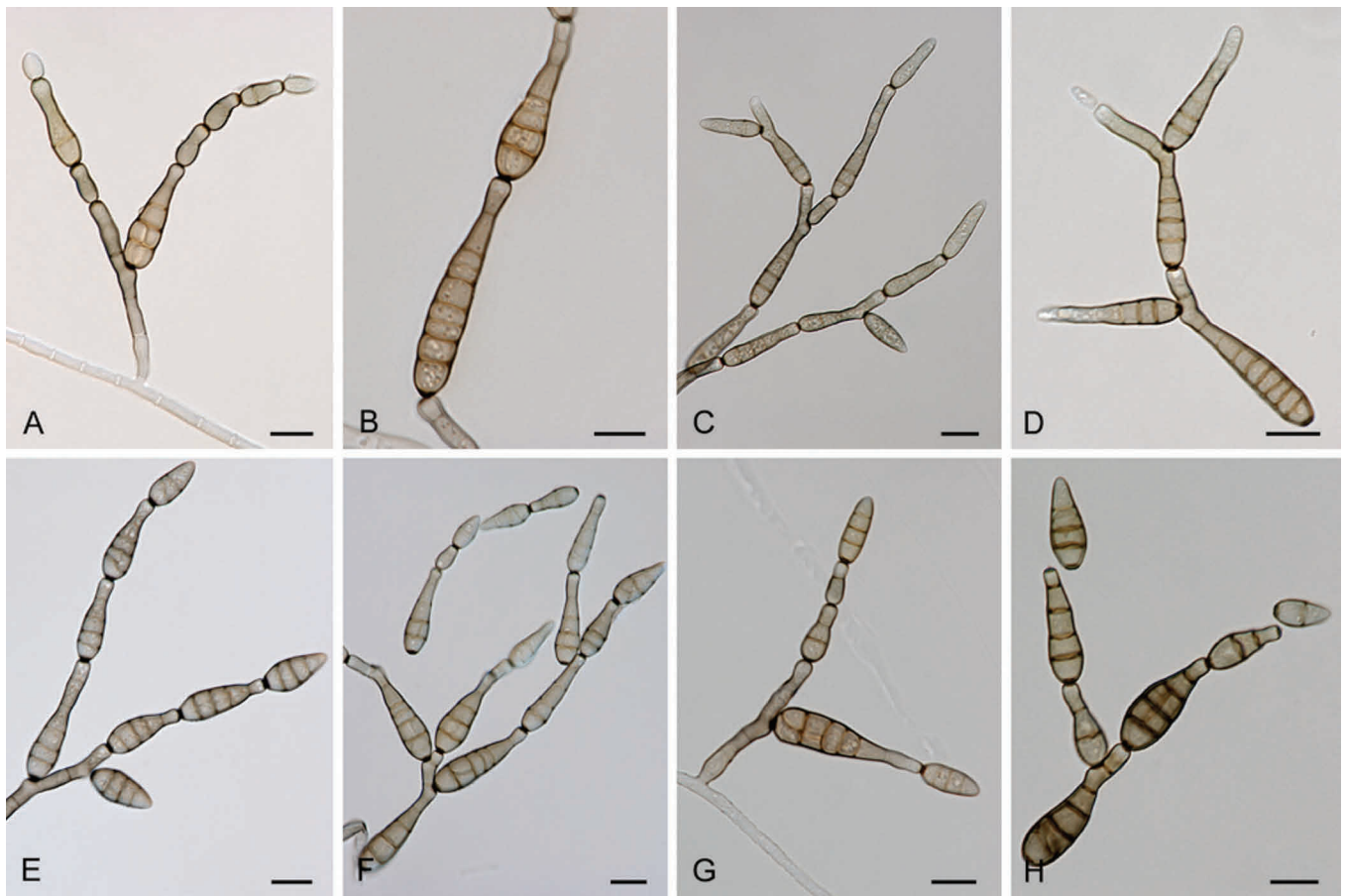
Fig. 14. Alternaria sect. Infectoriae : conidia and conidiophores. A–B. A. ethzedia . C–D. A. infectoria . E–F. A. conjuncta . G–H. A. oregonensis . Scale bars = 10 µm.
