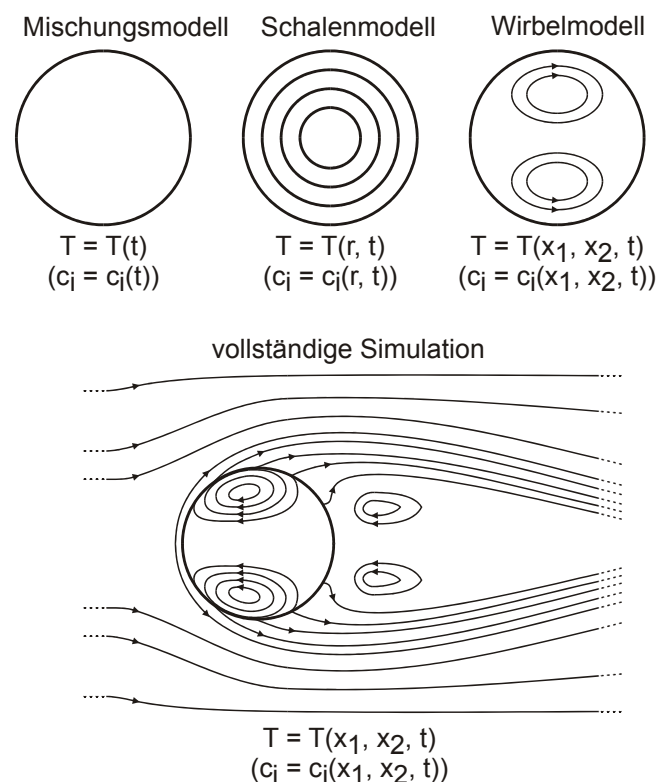
Abb. 2-3: Modellierungsansätze zur Tropfenverdrängung [SE1], [KLI]
