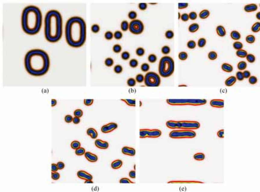
图 21 强分凝的两亲性线型ABC三嵌段高分子在溶液中的自组装形态 [66]
