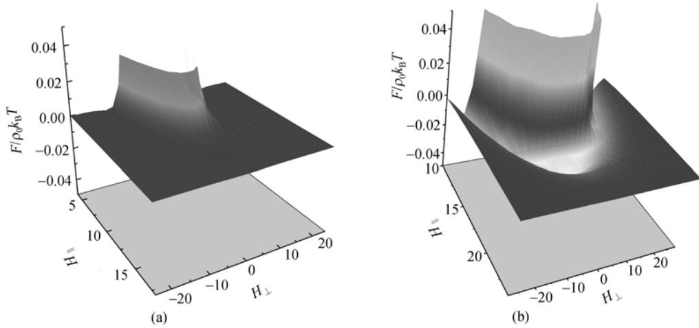
图 14 相互作用自由能密度随棒间距( H_{//} , H_{\perp} )的变化曲线与棒表面接枝密度的关系 N_{\alpha} = N_{\beta} = 50 , L = 31 , W = 3 . (a) \sigma = 0.039 , 不存在吸引势阱; (b) \sigma = 0.25 , 出现一个吸引势阱 [50]
