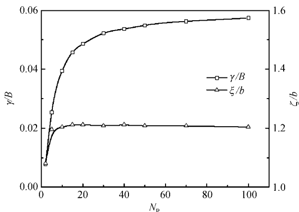
图 9 界面张力和界面宽度与高分子链长 N_p 的依赖关系 \chi_{ll}=5.0, \chi_{pl}=0 [41]
