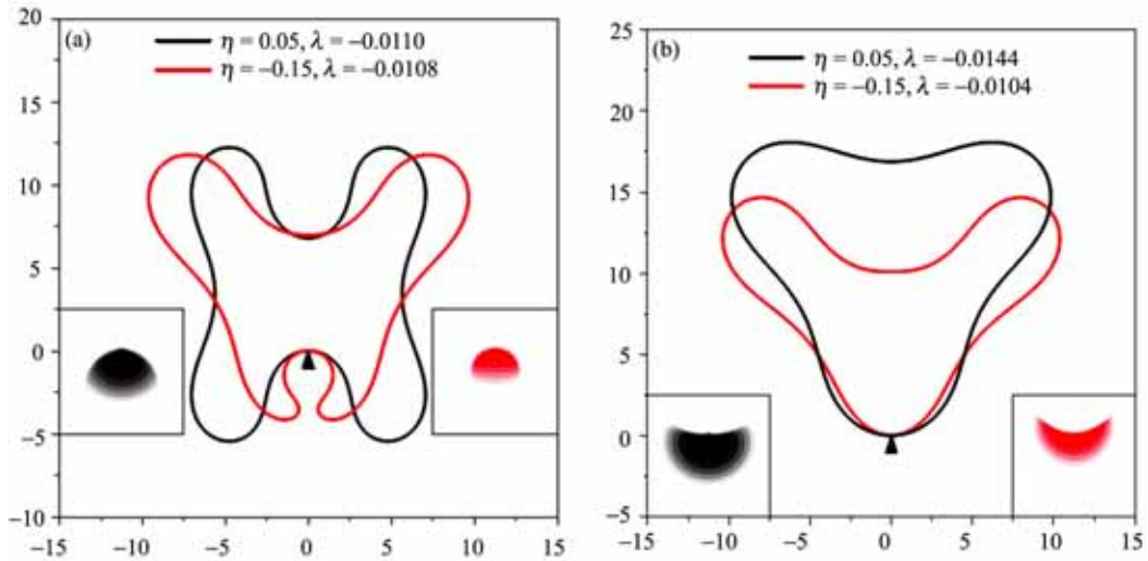
图 17 高分子链段与膜之间的相互作用参数对囊泡形状的影响 图中的囊泡形状是三维柱对称旋转体的截面
