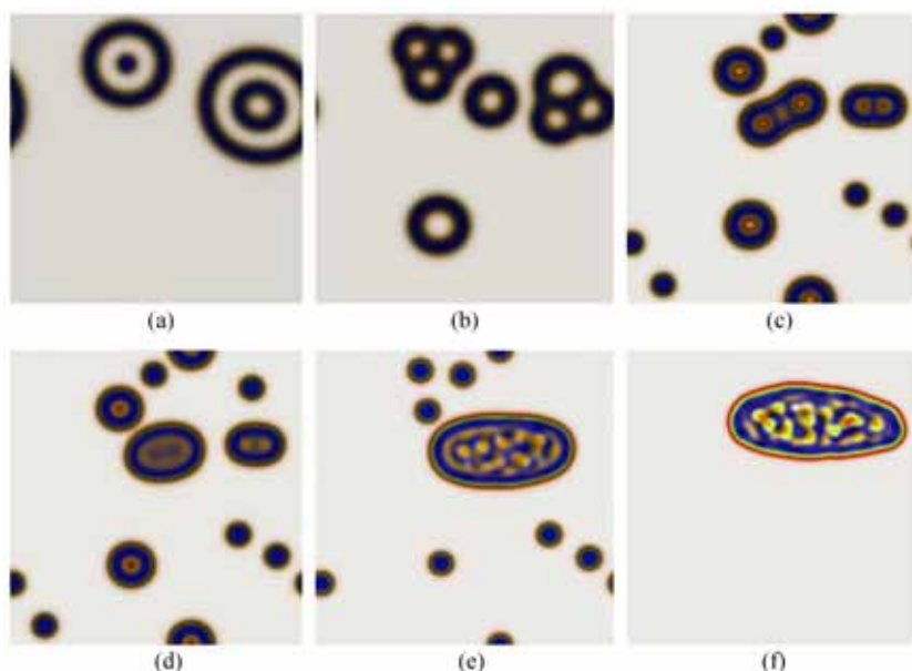
图 20 弱分凝的两亲性ABC线型三嵌段高分子在溶液中的自组装形态 [66]
