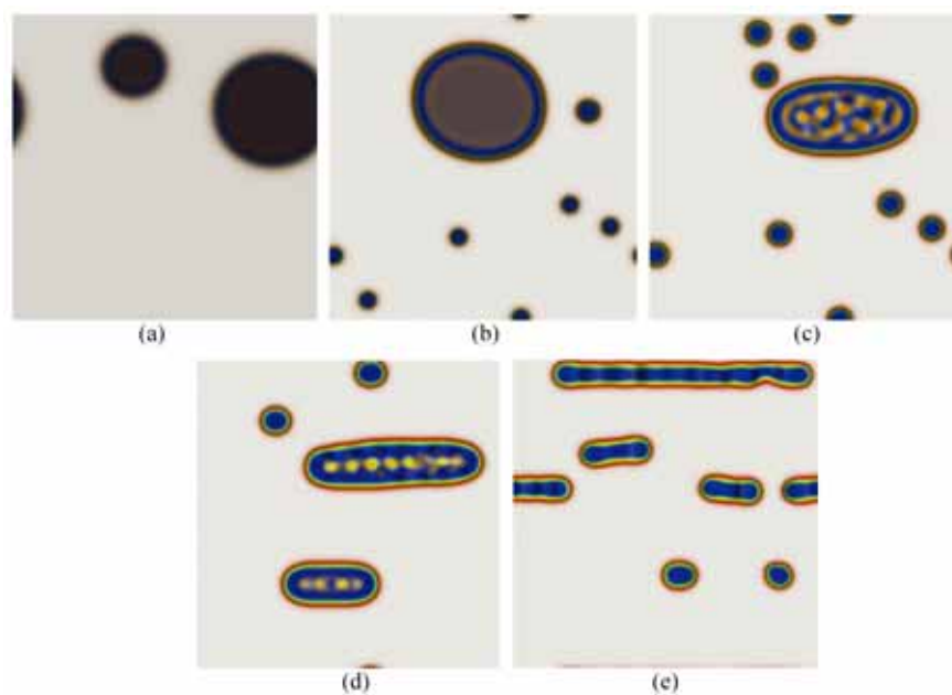
图 22 弱分凝的两亲性线型ABC三嵌段高分子, 当中间嵌段B强疏水时, 随嵌段C的不同疏水程度在溶液中的自组装形态 [66]
