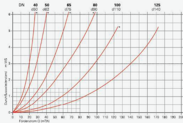
Rückspülventile - Druckverlustkurve
