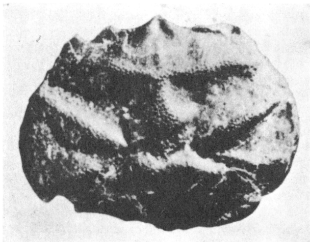
TEXT-FIG. 1. Costacopluma senegalensis (Remy). Holotype, \times 2 . Reproduced from Bull. Soc. géol. Fr. (7) 1, pl. 19a, fig. 1, with the kind permission of the Société géologique de France.
