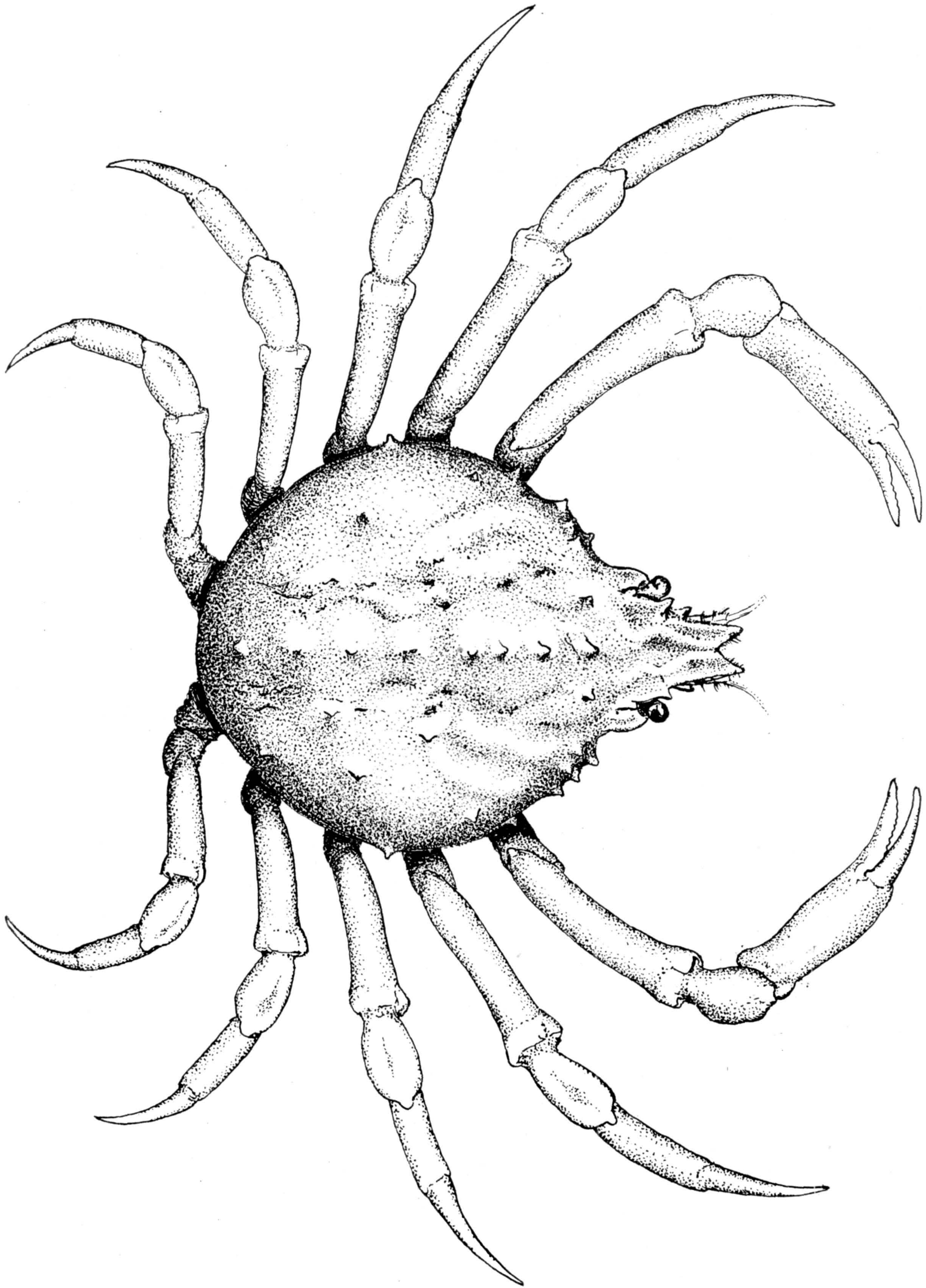
LIBINIA SETOSA. (PAGE 327)
