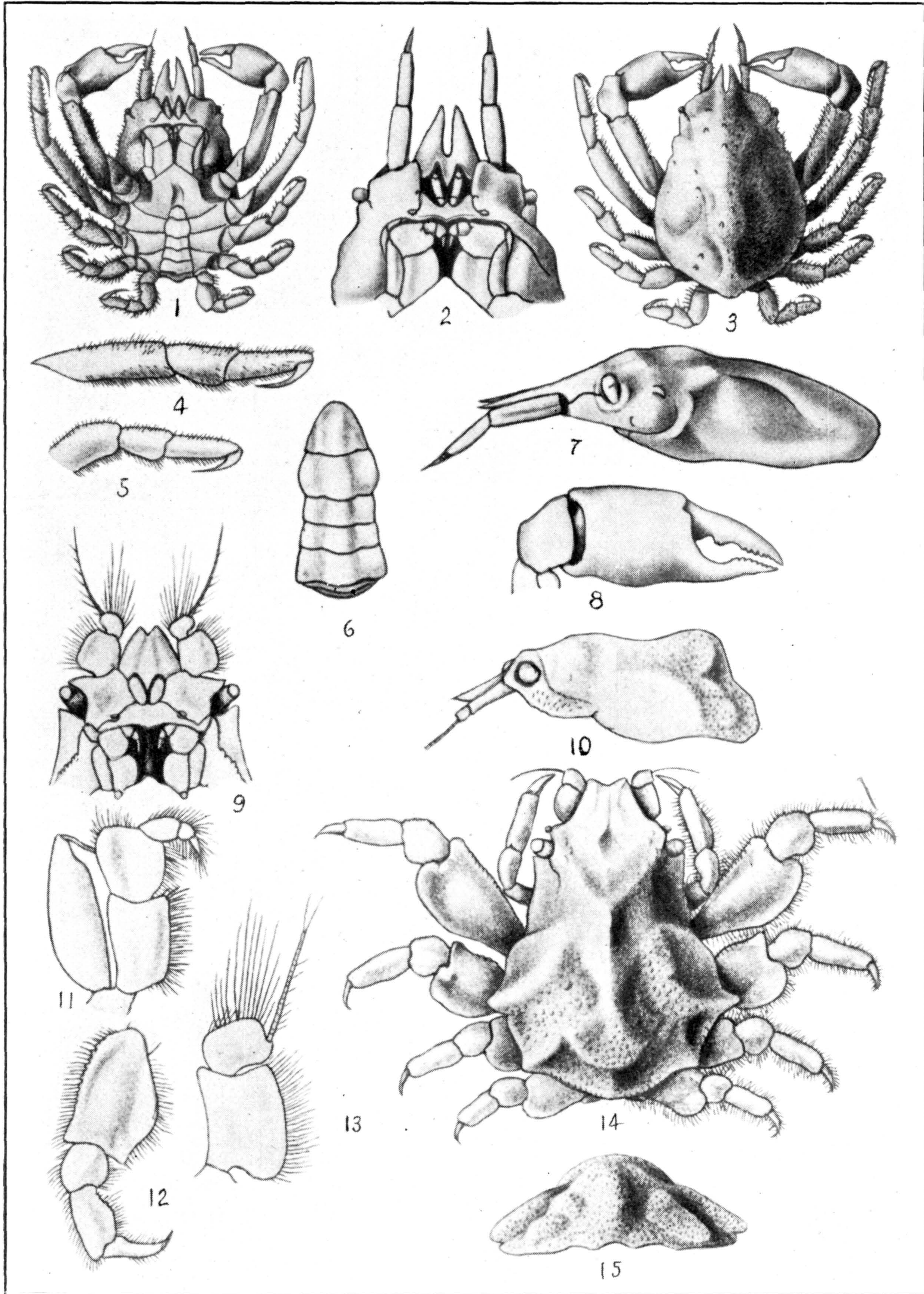
1-8. Thersandrus compressus . (PAGE 343.) 9-15. Hemus cristulipes . (PAGE 345)
