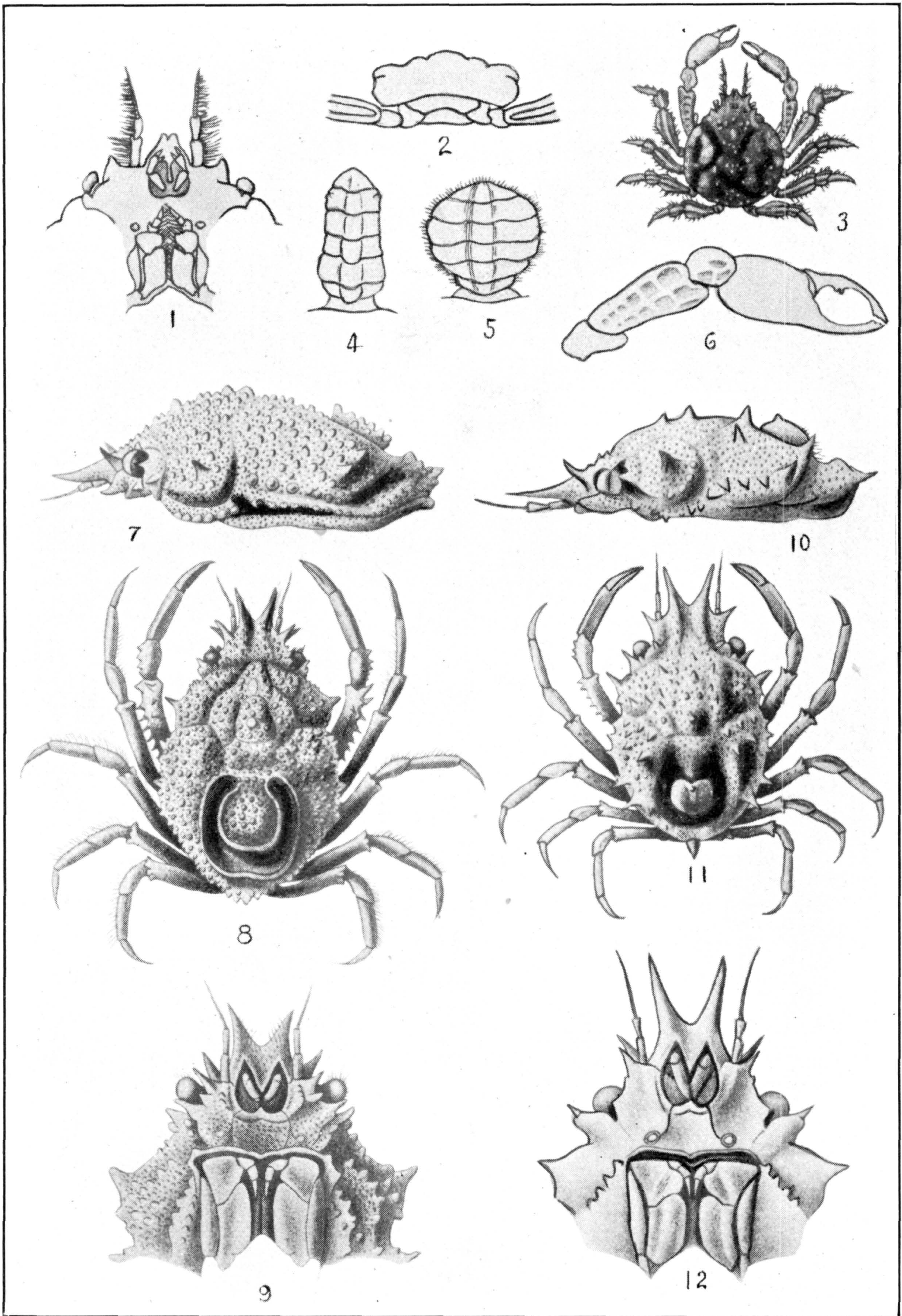
1-6. THOE EROSA . (PAGE 351.) 7-9. TEMNONOTUS GRANULOSUS . (PAGE 341.) 10-12. T. SIMPLEX . (PAGE 342)
