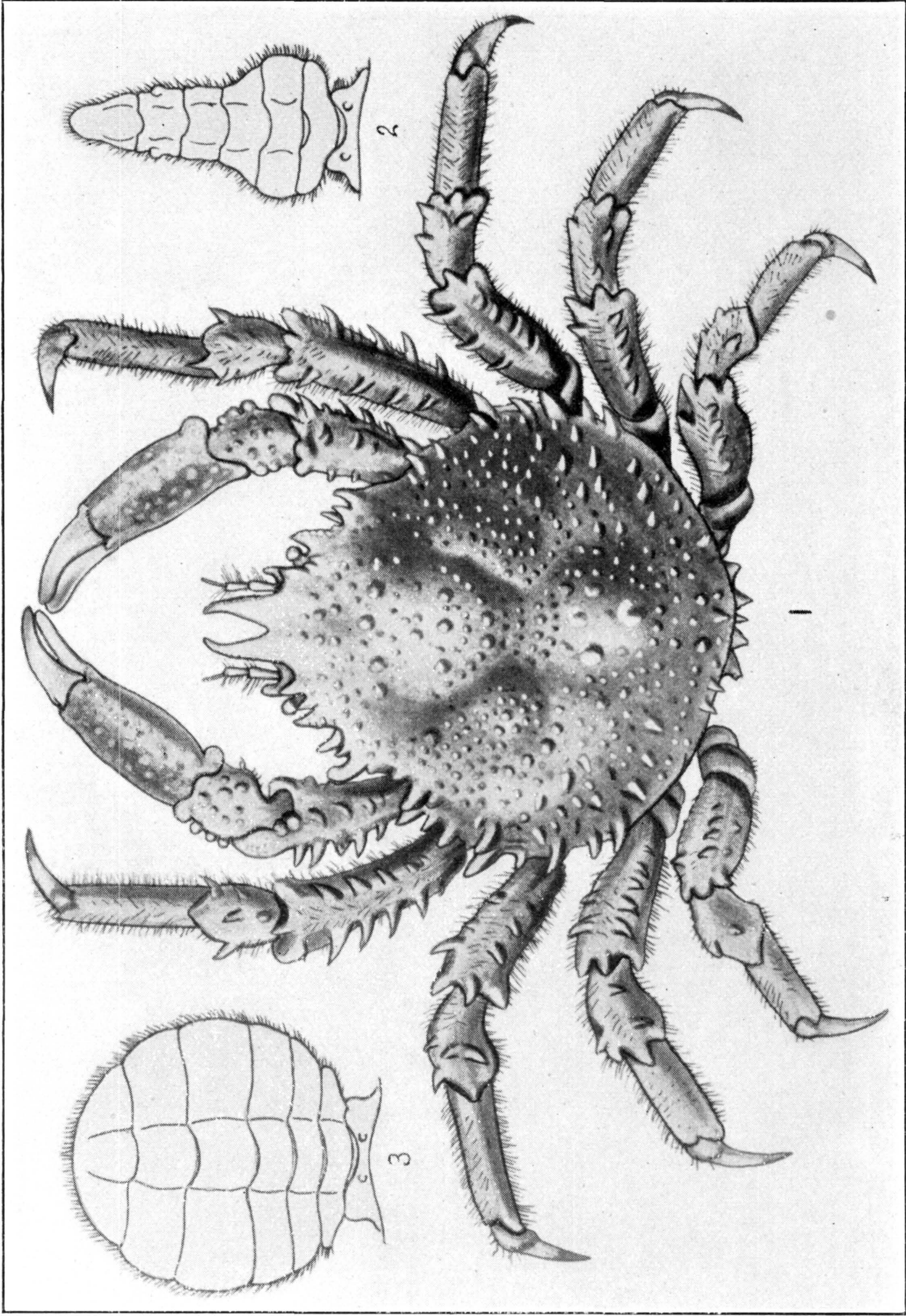
MITHRAX ROSTRATUS. (PAGE 386)
