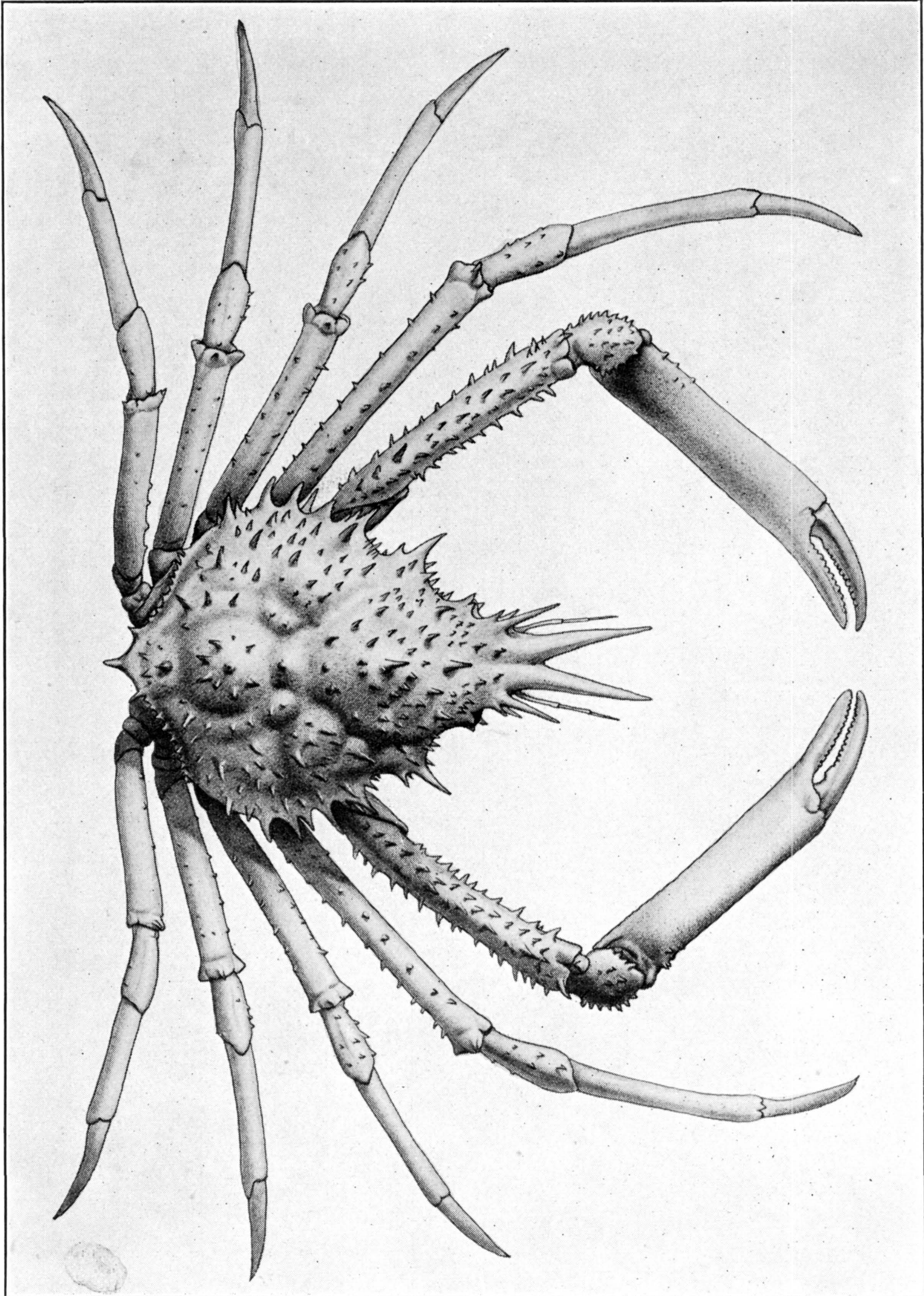
NIBILIA ANTILOCAPRA. (PAGE 290)
