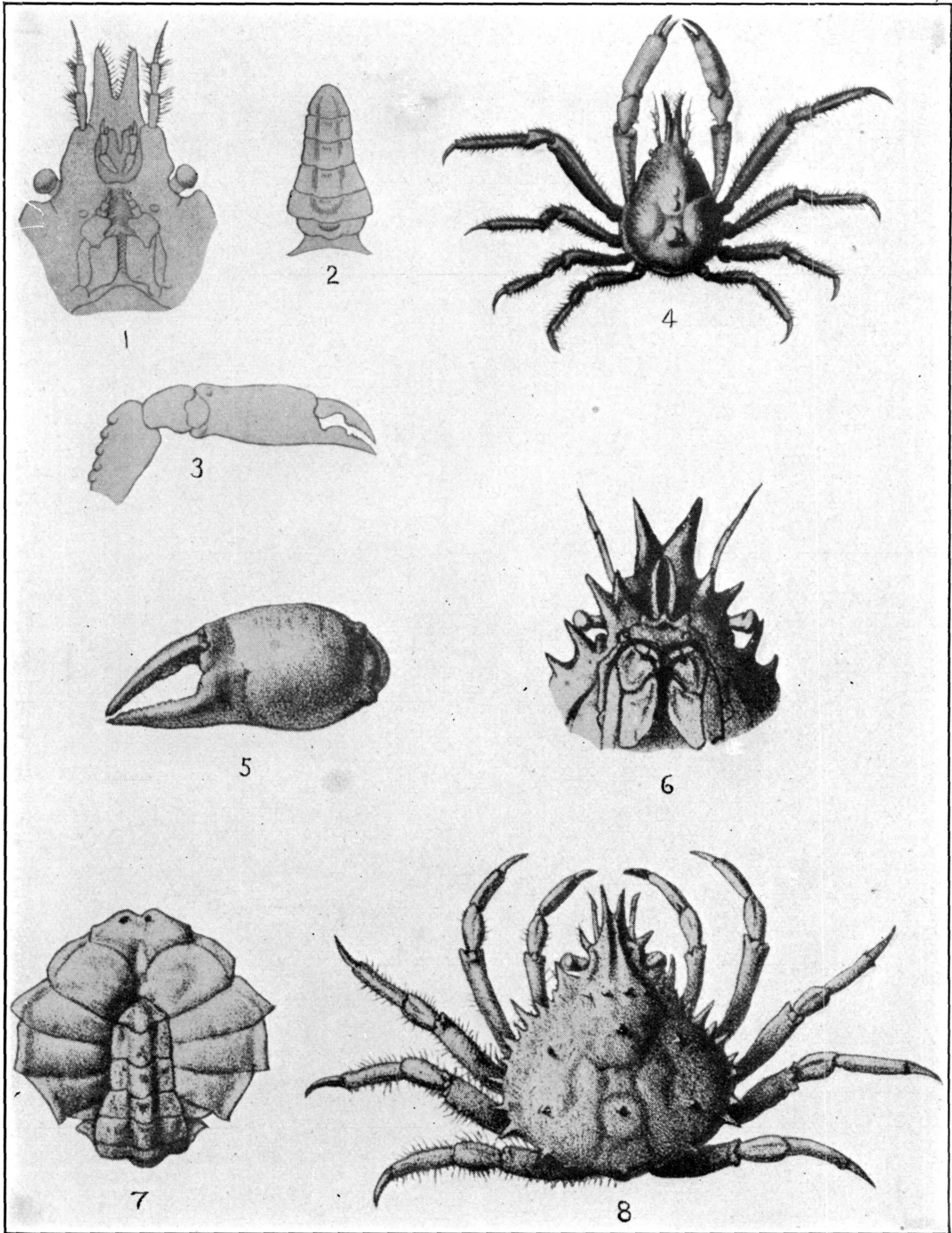
1-4. PELIA PULCHELLA. (PAGE 284.) 5-8. MICROPISA VIOLACEA. (PAGE 303)
