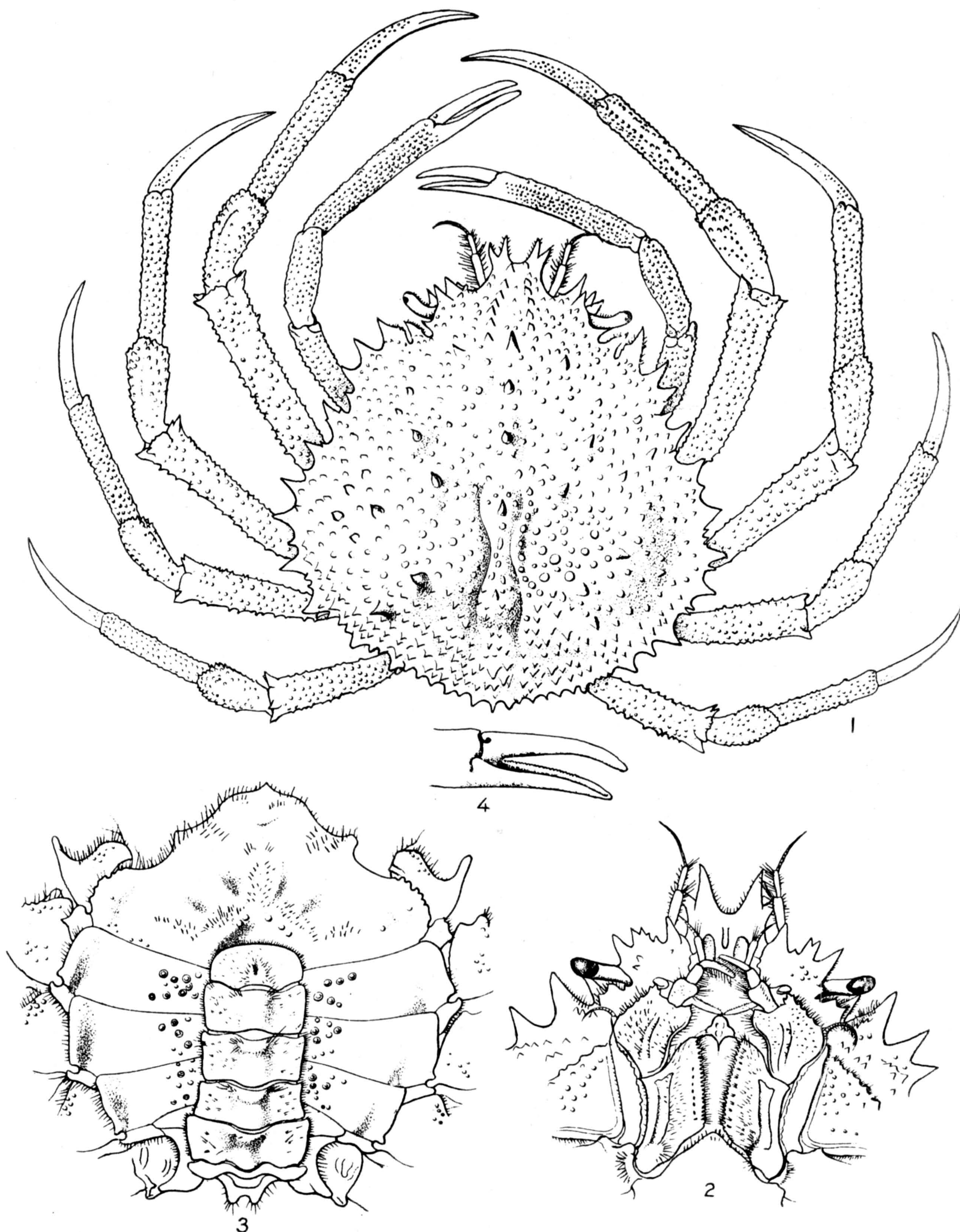
MAIOPSIS PANAMENSIS. (PAGE 338)
