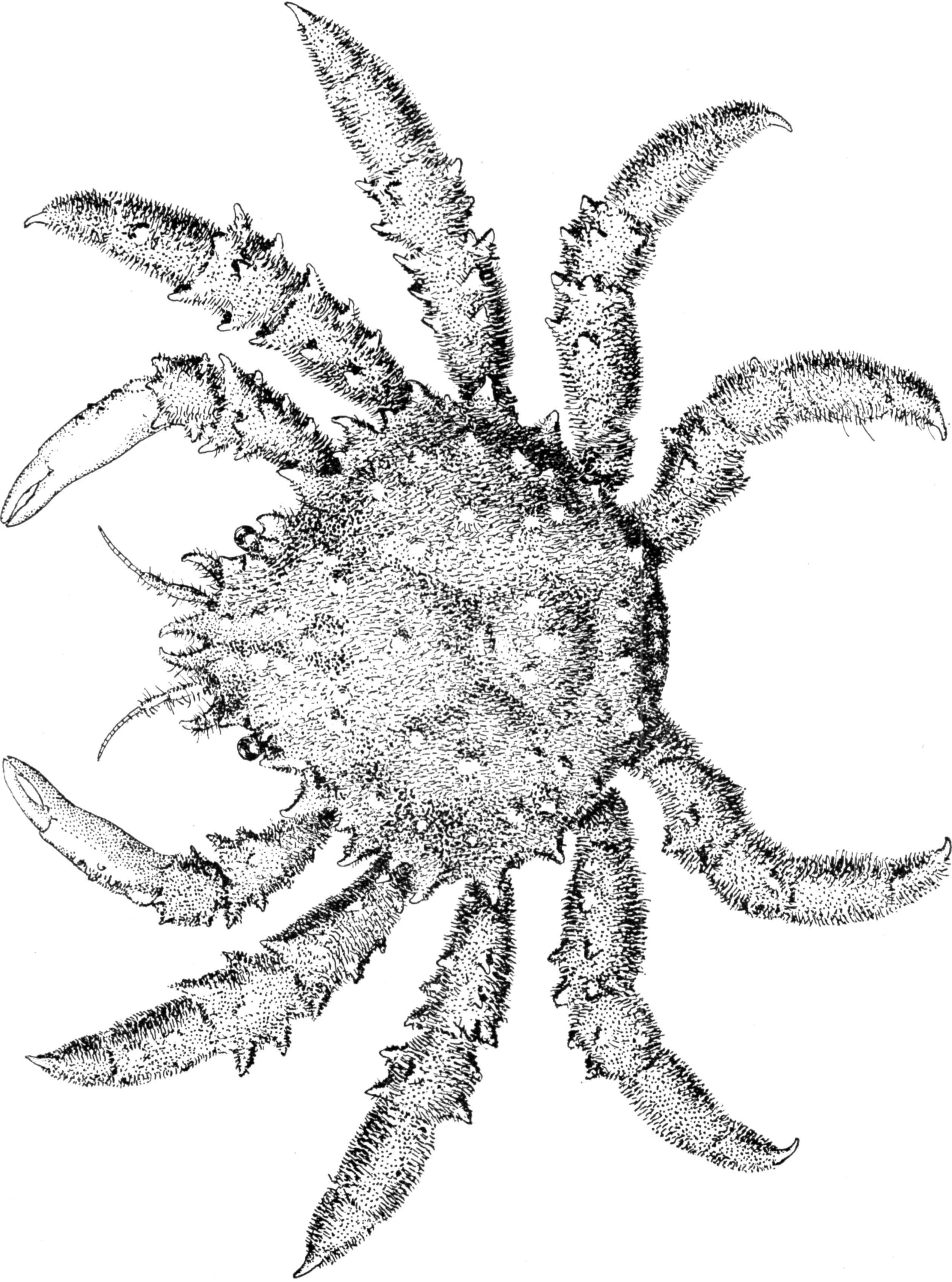
MITHRAX PILOSUS. (PAGE 394)
