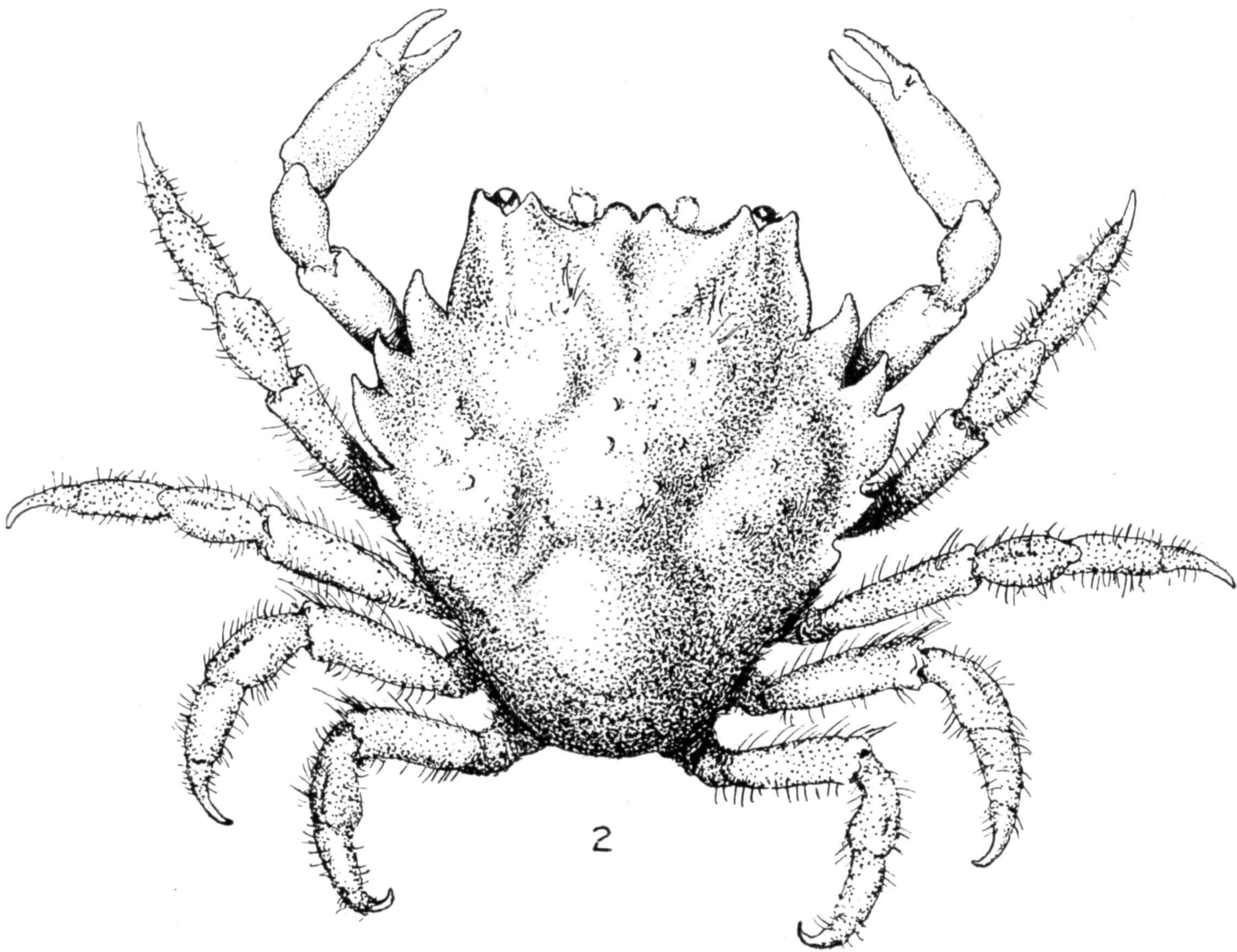
1. PITHO PICTETI. (PAGE 359.) 2. P. LHERMINIERI. (PAGE 362)
