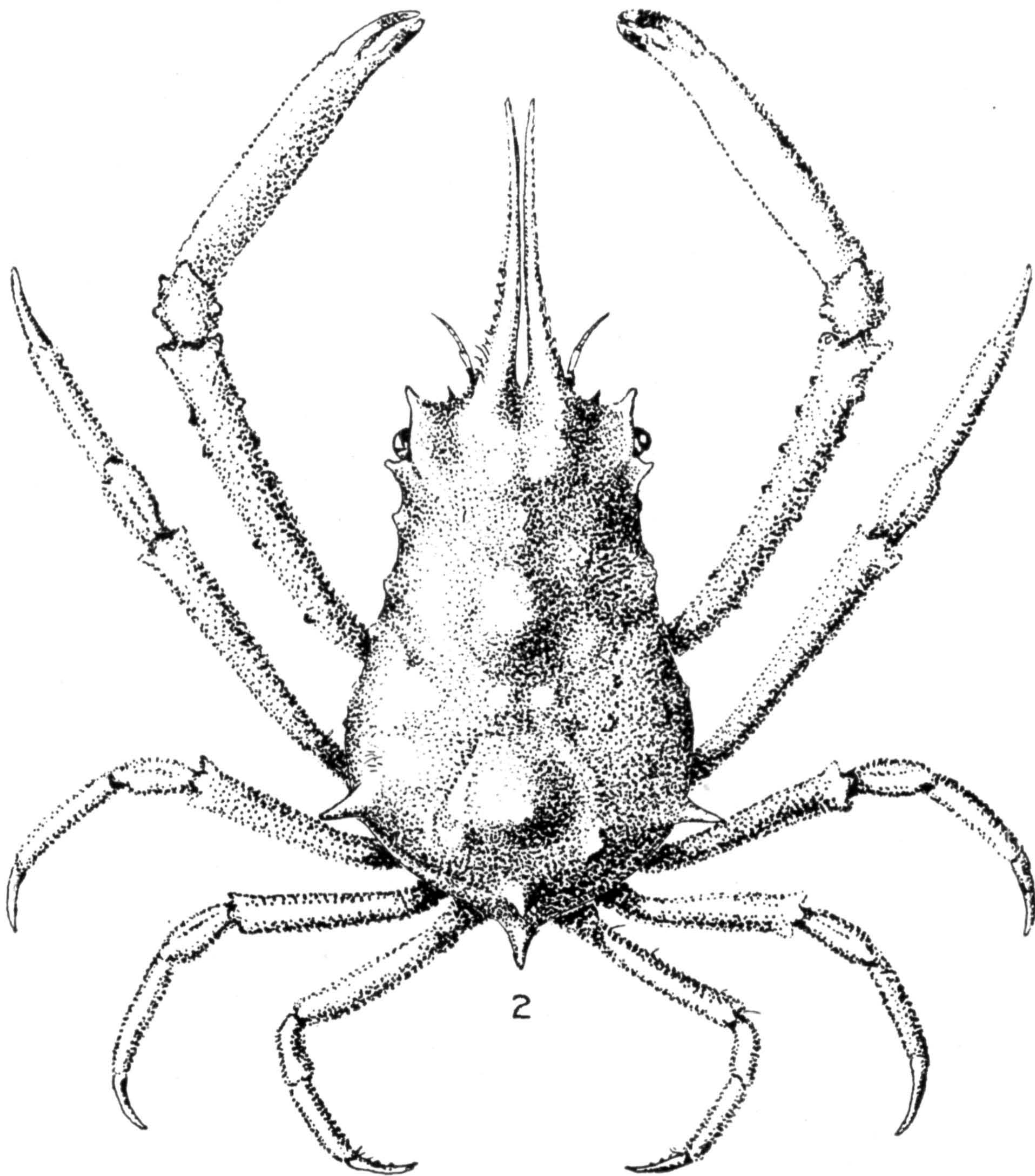
1. PITHO MIRABILIS. (PAGE 366.) 2. LEPTOPISA SETIROSTRIS. (PAGE 375)
