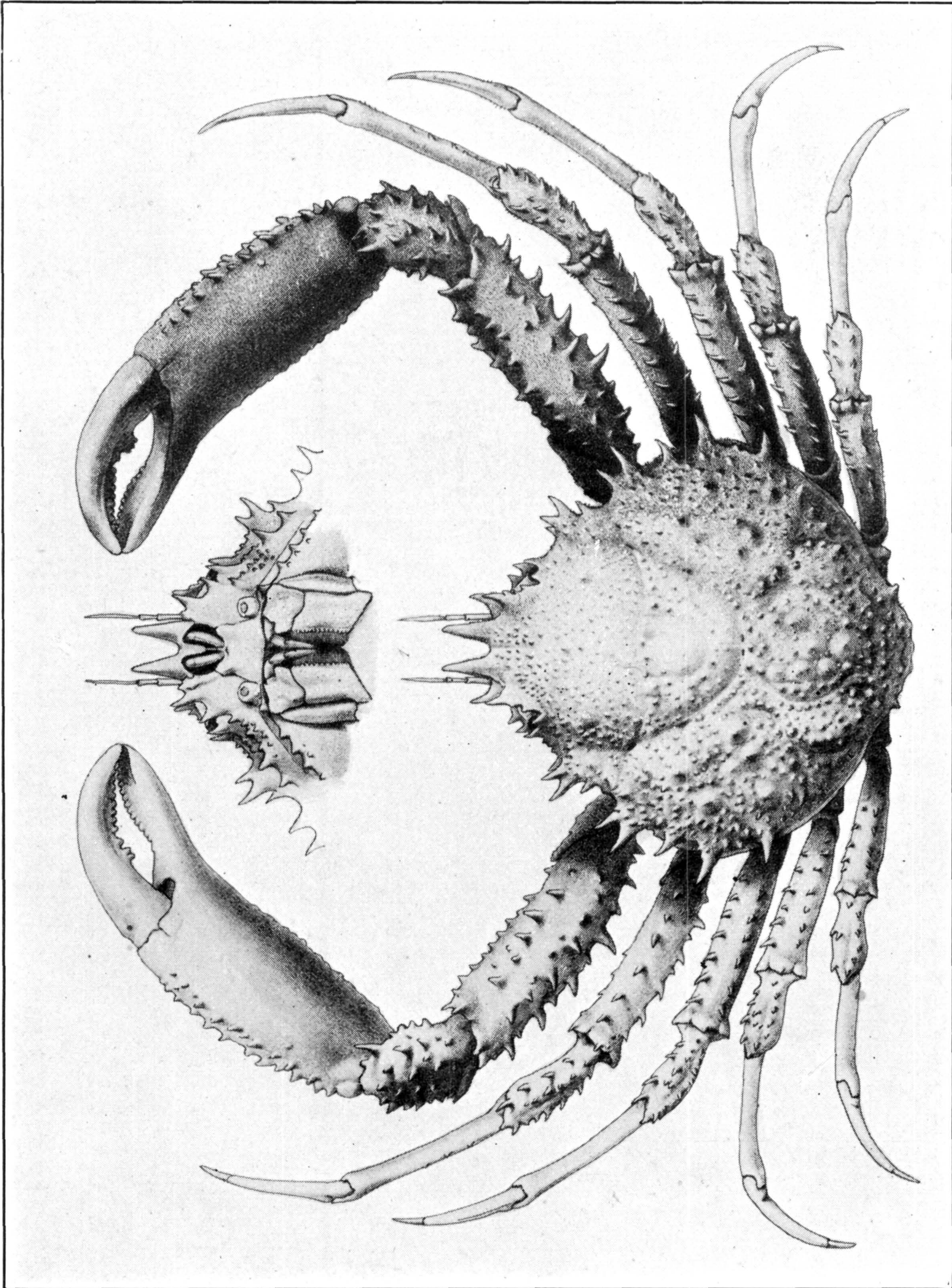
MITHRAX CORNUTUS. (PAGE 386)
