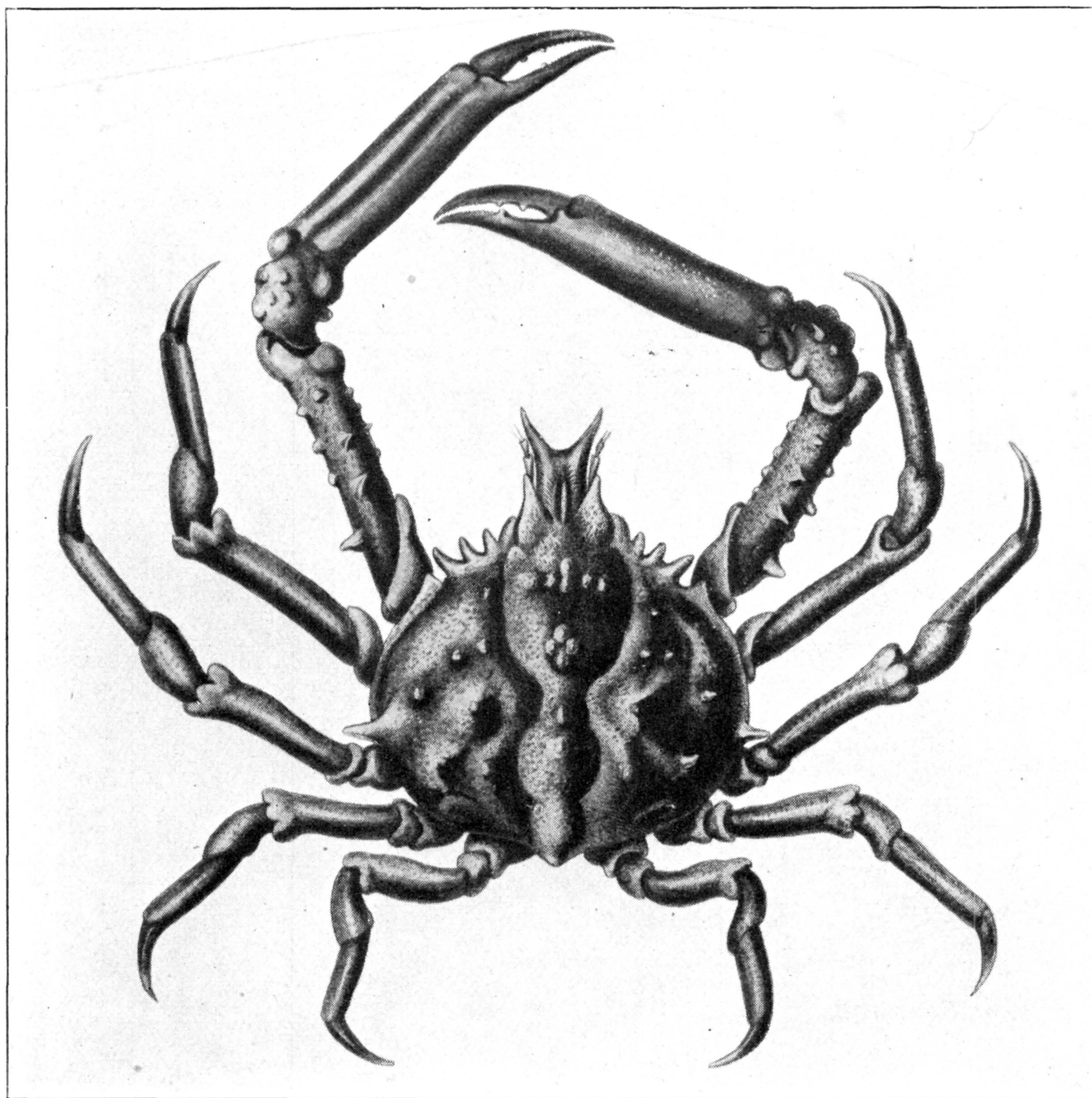
LIBINIA ROSTRATA. (PAGE 329)
