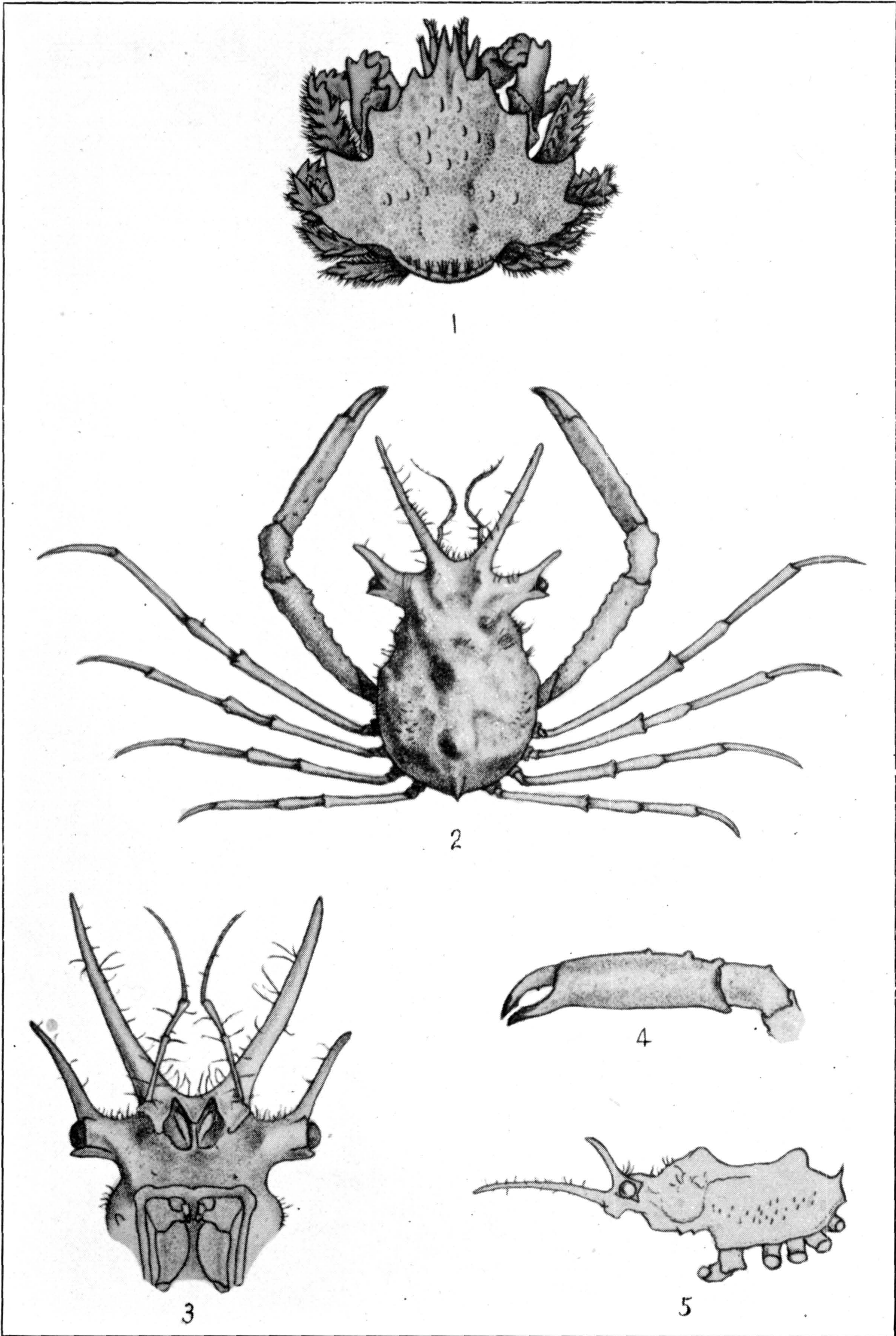
1. ANAPTYCHUS CORNUTUS. (PAGE 378.) 2-5. PICROCEROIDES TUBULARIS. (PAGE 354)
