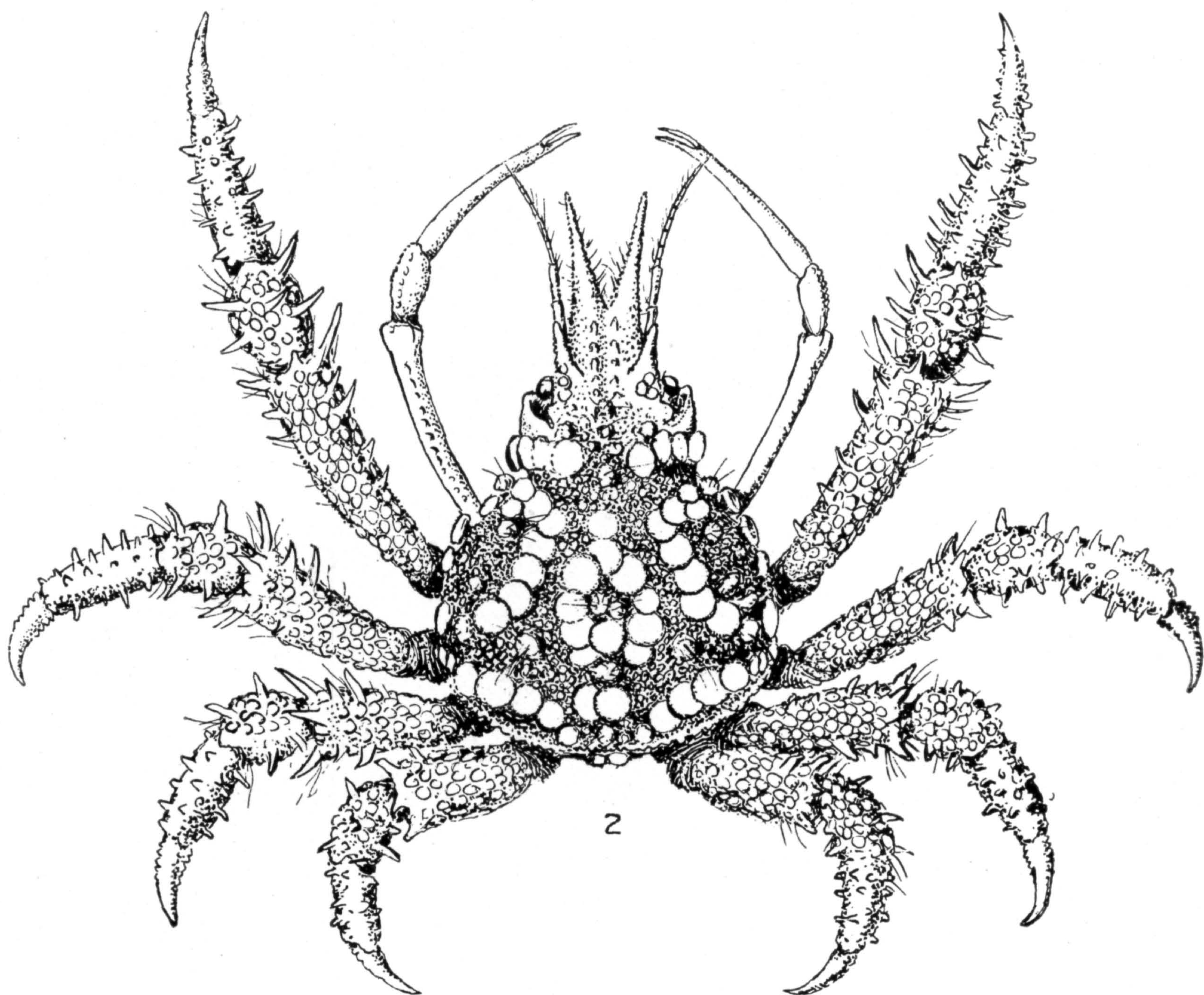
1. LIBINIA MEXICANA . (PAGE 328.) 2. LEPTECES ORNATUS . (PAGE 292)
