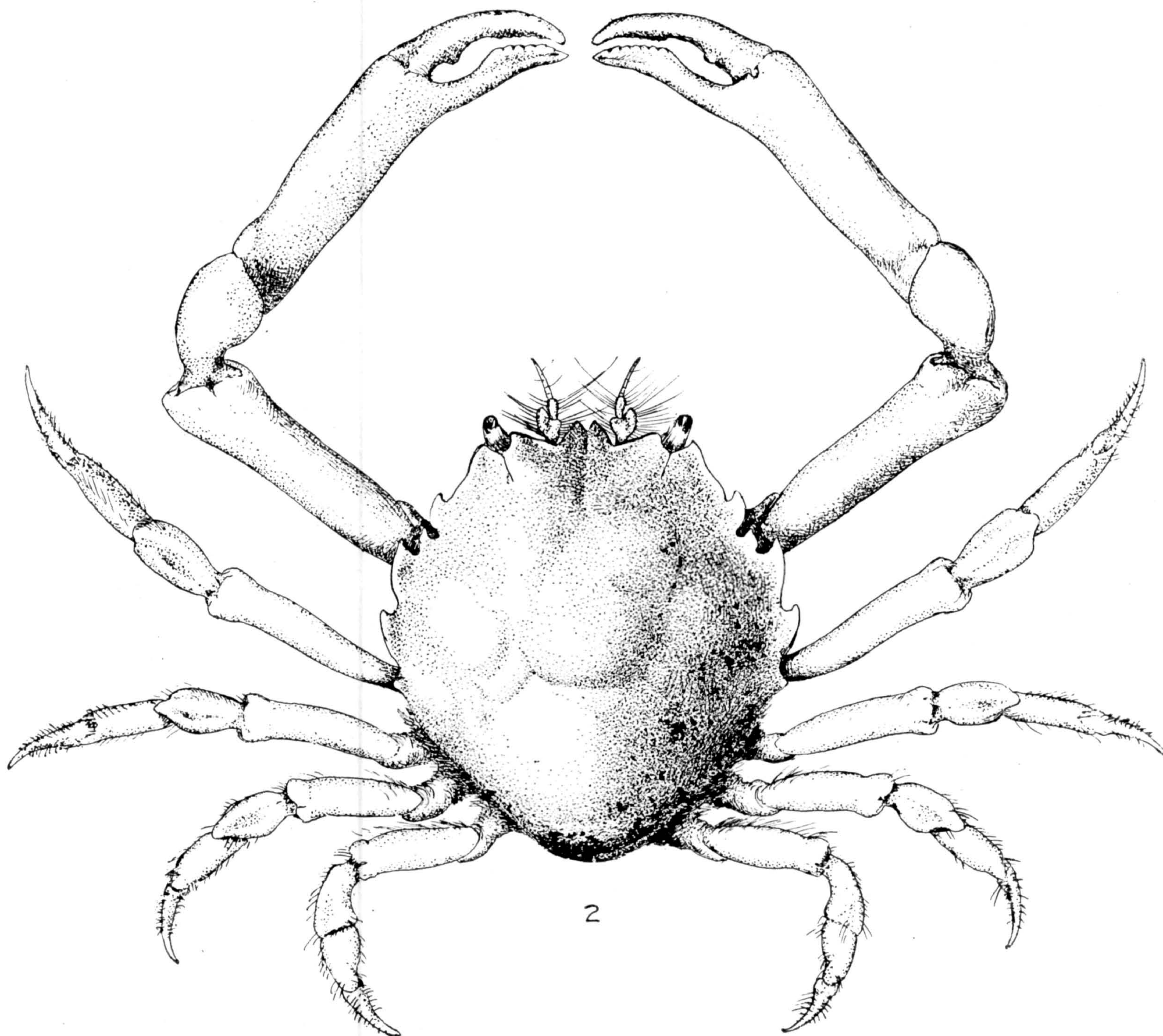
1. PITHO ACULEATA . (PAGE 357.) 2. P. ANISODON . (PAGE 368)
