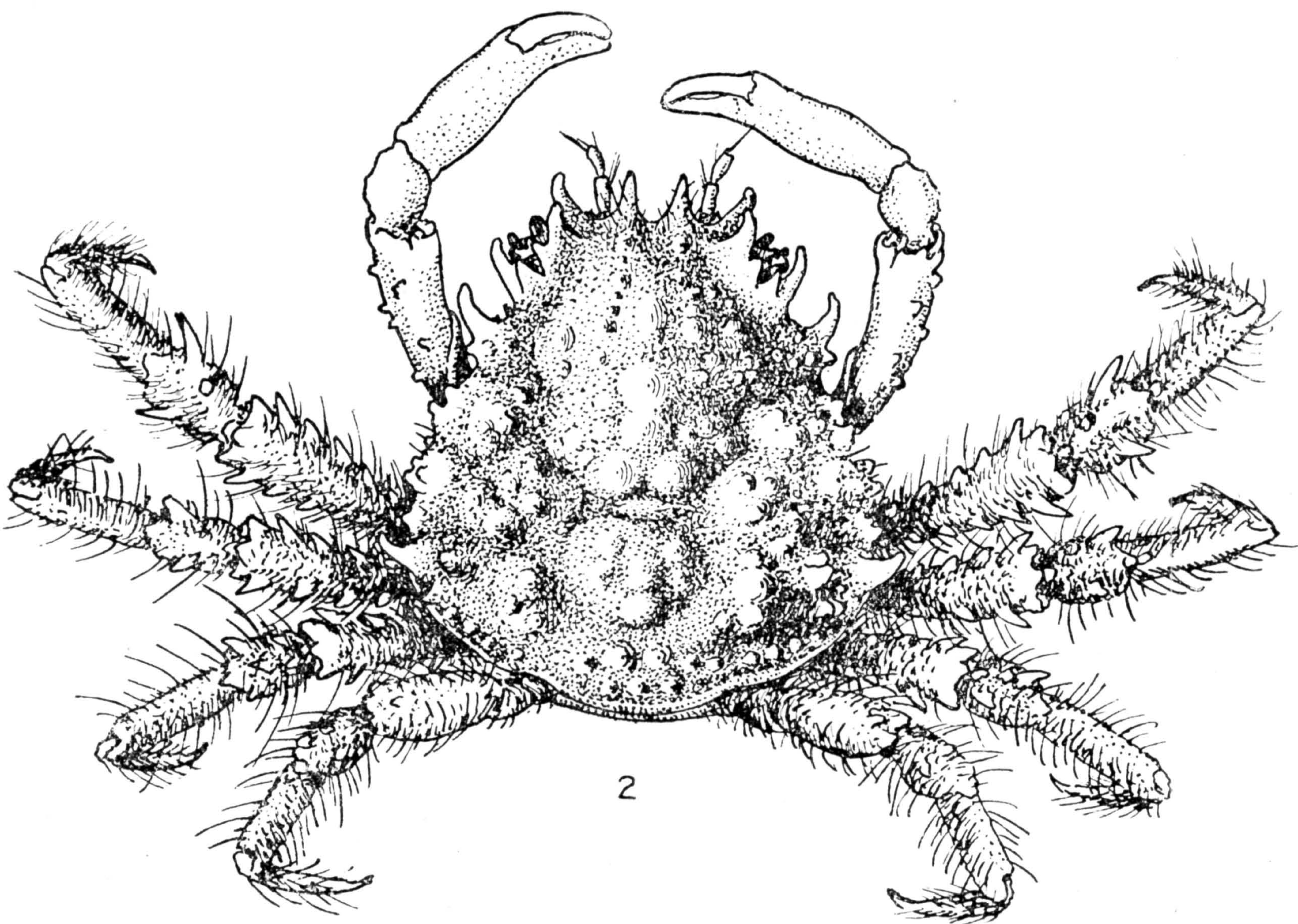
1. MITHRAX ACUTICORNIS. (PAGE 388.) 2. M. HOLDERI. (PAGE 392)
