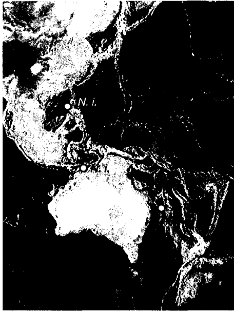
FIG. 9. — Carte bathymétrique de l'Ouest Pacifique faisant apparaître les grands reliefs sous-marins, fosses, rides, arc d'îles. Abréviations: N. i. , Neoglyphea inopinata ; N. n. , Neoglyphea neocaledonica n. sp. (fond de carte du NOAA, http://www.ngdc.noaa.gov ).
