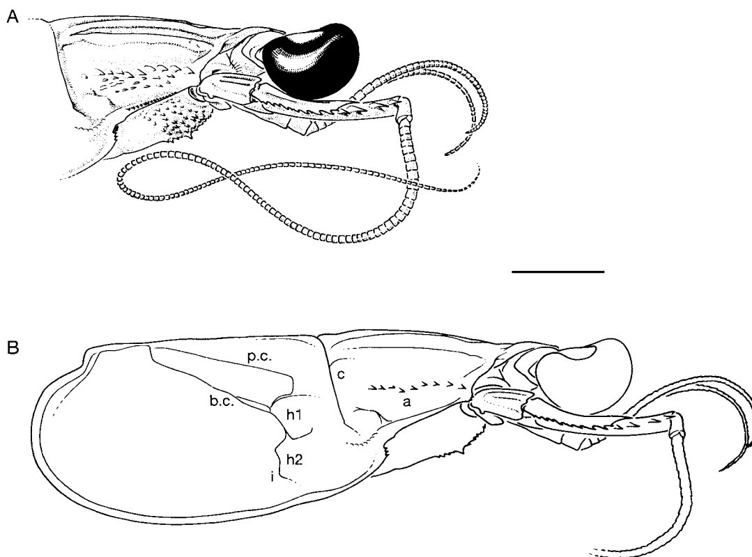
FIG. 4. — Neoglyphea neocaledonica n. sp., holotype : A , vue latérale de la partie du corps en avant du sillon cervical ; B , céphalothorax en vue latérale montrant la disposition des sillons. Abréviations : a , sillon antennaire ; b.c. , sillon branchiocardiaque ; c , sillon cervical ; h1 , h2 , sillons hépatiques ; i , sillon inférieur ; p.c. , sillon post-cervical. Échelle : 5 mm.
