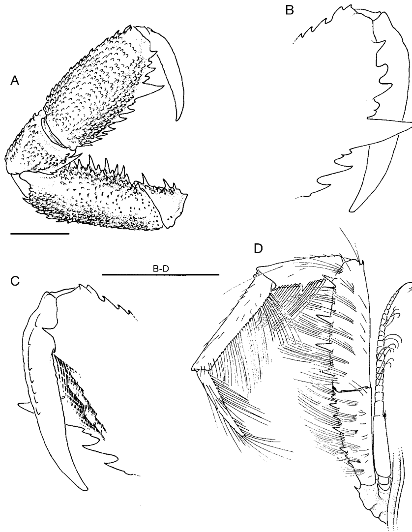
FIG. 6. — Neoglyphea neocaledonica n. sp., holotype: A-C , premier périopode droit; A , entier; B, C , détail de la pseudo-pince, faces externe ( B ) et interne ( C ); D , troisième maxillipède gauche, face externe. Échelles: 5 mm.
