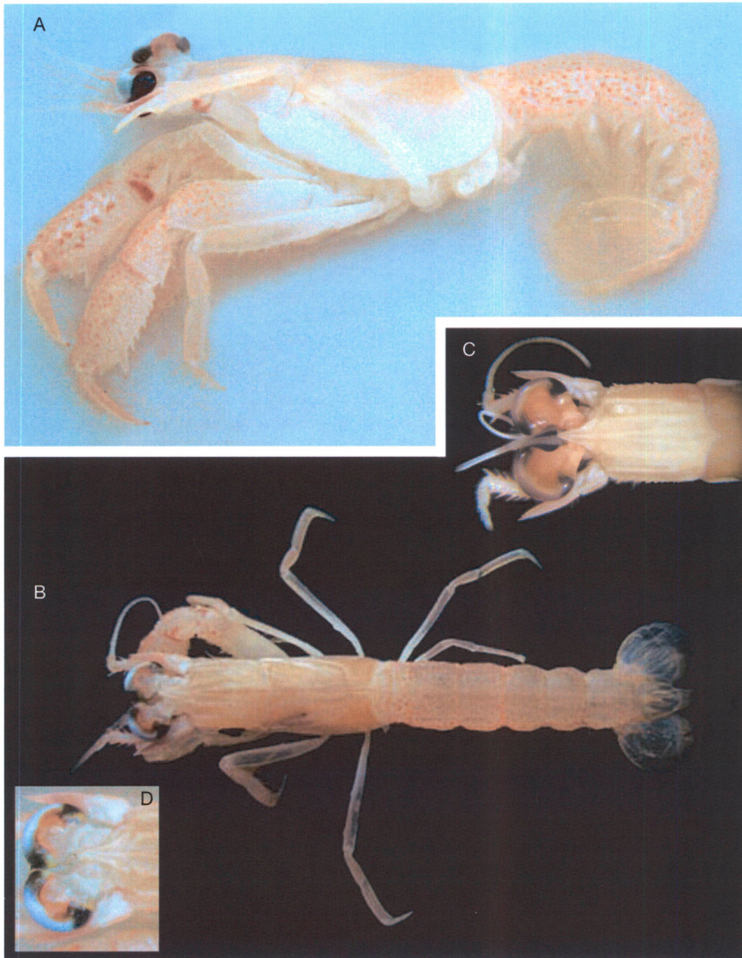
FIG. 2. — Neoglyphea neocaledonica n. sp., holotype photographié sur le vivant, quelques minutes après sa capture (à l'exception de la figure C, faite plus tardivement) : A , vue latérale de l'animal entier ; B , vue dorsale de l'animal entier ; C , vue dorsale de la partie antérieure du corps ; D , coloration des yeux (photos J. Lai).
