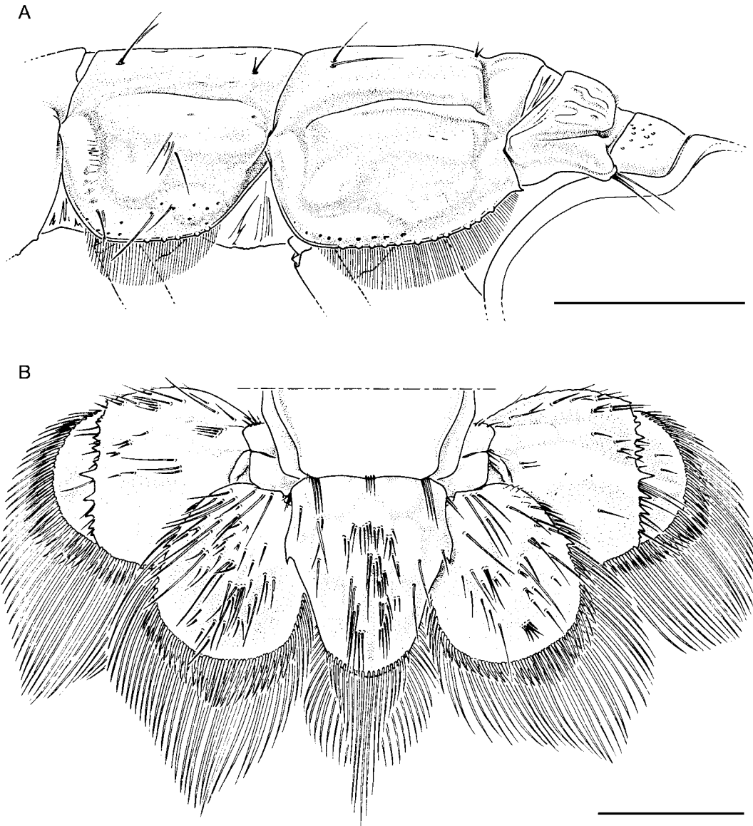
FIG. 7. — Neoglyphea neocaledonica n. sp., holotype: A, vue latérale de la partie antérieure droite de l'abdomen (segments 1-3); B, telson et uropodes. Échelles: 5 mm.
