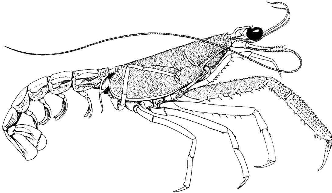
FIG. 1. — Neoglyphea inopinata Forest & de Saint Laurent, 1975, ♀, 115 mm, Philippines, vue latérale (d'après Forest et de Saint Laurent 1989).
