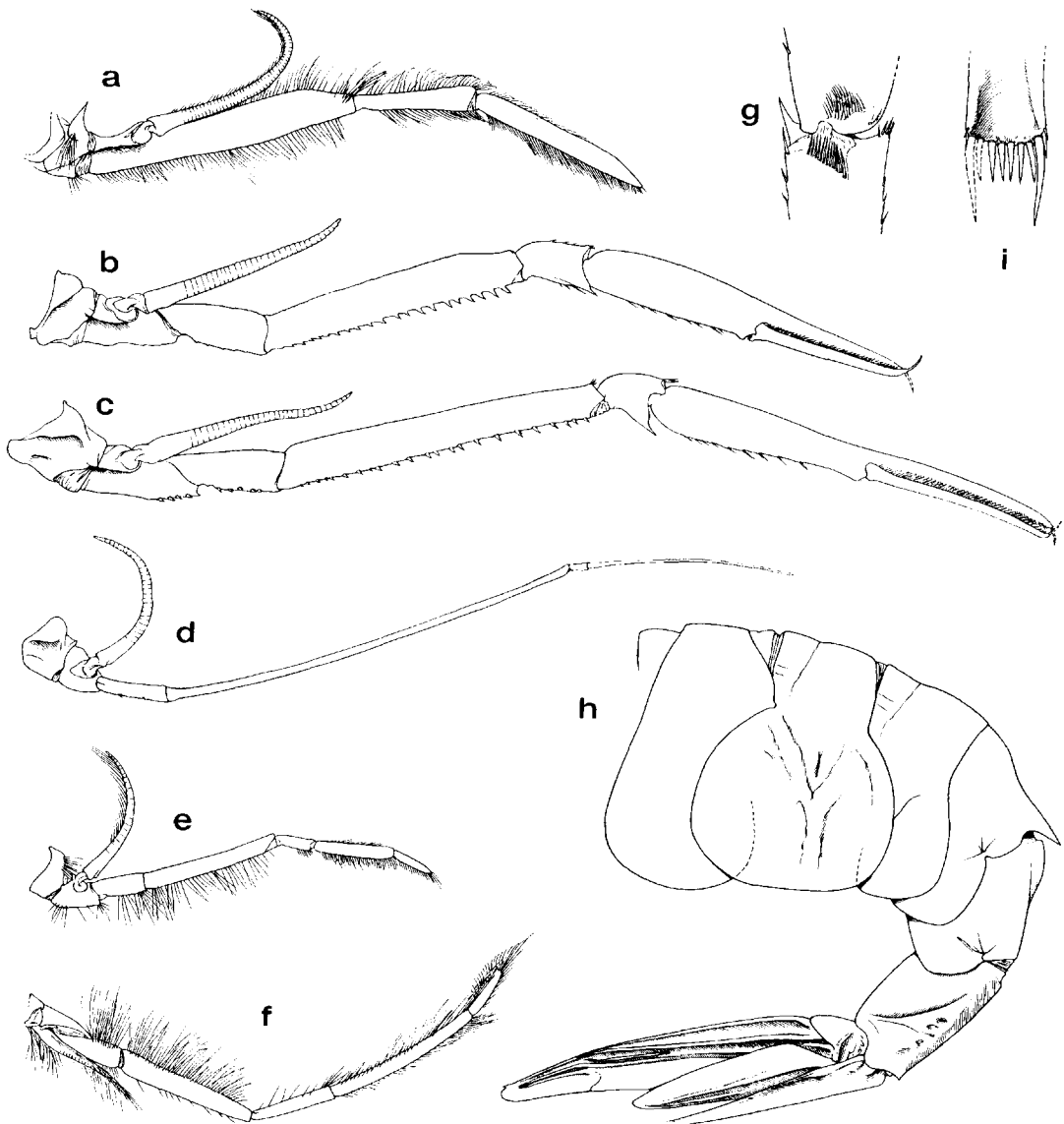
FIG. 4. -- Eupasiphae paucidentata sp. nov., ♀ ov. holotype 34,0 mm, Madagascar (MP-Na 12530) : a, troisième maxillipède droit ; b, premier péréiopode droit ; c, deuxième péréiopode droit ; d, troisième péréiopode droit ; e, quatrième péréiopode droit ; f, cinquième péréiopode droit ; g, extrémité du carpe et base du propode du premier péréiopode droit, face interne ; h, abdomen, vue latérale ; i, extrémité du telson, vue dorsale. Les figures a-f sont à la même échelle.
