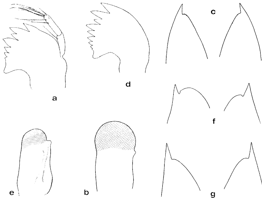
FIG. 5 a. Eupasiphae gilesii (Wood Mason, 1892), ♂ 14,8 mm, Madagascar (MP-Na 12533) : mandibule gauche. FIG. 5 b-c. Eupasiphae paucidentata sp. nov., ov. holotype 34,0 mm, Madagascar (MP-Na 12530) : b, œil gauche vu dans le plan du tubercule du bord interne ; c, extrémité des scaphocérites. FIG. 5 d-g. Eupasiphae serrata (Rathbun, 1902) : d-f, ♀, ov. 34,0 mm, Atlantique oriental (MP-Na 12529) : d, mandibule gauche ; e, œil gauche vu dans le plan du tubercule du bord interne ; f, extrémités des scaphocérites. — g, ♀ 28,5 mm, holotype de Parapasiphae grimaldii Coutière, Atlantique oriental (MP-Na 1818) : extrémités des scaphocérites.
