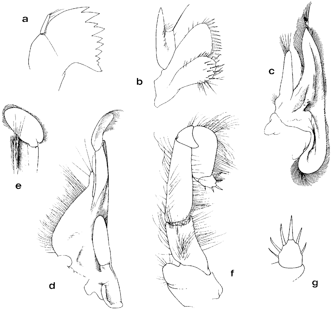
FIG. 3. — Eupasiphae paucidentata sp. nov., ♀ ov. holotype 34,0mm, Madagascar (MP-Na 12530) : a, mandibule droite, face ventrale; b, maxillule droite, face ventrale; c, maxille droite, face dorsale; d-e, premier maxillipède droit, face dorsale et extrémité en vue externe; f-g, deuxième maxillipède, face ventrale et dactyle en plan. Les figures a-d et f sont à la même échelle.
