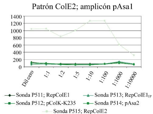
Figura suplementaria 3.2.H. Validación de las sondas MOB P5 para el array en suspensión. Las magnitudes son las mismas que en casos anteriores. Las curvas de validación de las sondas P512 y P514 no se hicieron por falta de controles positivos.
