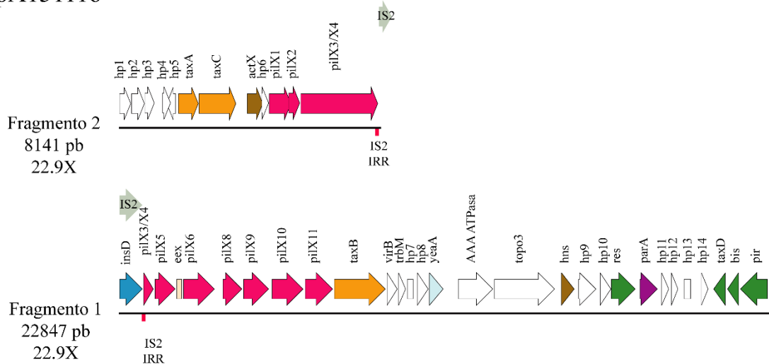
Figura 3.4.F. Mapa genético del plásmido (incompleto) pA13111o. La leyenda es igual que en la figura 3.3.A.
