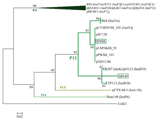
Figura 3.3.F. Filogenia de la subfamilia MOB_{P12} añadiendo las relaxasas de aislados IncB/O. Esta filogenia se ha reconstruido como ya se ha indicado (Sección 2) salvo que aquí hemos utilizado únicamente el fragmento amplificado por las correspondientes sondas DPMT (de unos 51 aminoácidos de longitud) de manera que la topología de la misma puede variar respecto a la presentada en la figura 3.1.B. Los otros cluster dentro de MOB_{P1} aparecen comprimidos por claridad, aportándose ejemplos representativos contenidos en ellos. Las nuevas relaxasas aparecen recuadradas en verde. Más información sobre MOB_{P1} en la figura 3.1.B.
