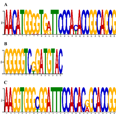
Figura 3.5.K. Logo del iterón consenso de los plásmidos MOB F112 / IncN-like . Se predijeron, como ya se ha descrito, las secuencias y el número de iterones de los replicones de los A) plásmidos MOB F112 / IncN4 detallados en el texto, comparados con los logos de los plásmidos B) MOB F112 / IncN3 pN-Cit y C) MOB F112 / IncN1 R46. Las alturas de cada base responden a su frecuencia.
