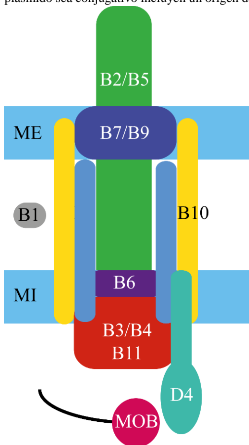
Figura 1.C. Organización del T4SS de A. tumefaciens . La secuencia de ensamblado y la función de todas las proteínas representadas en esta figura se detallan en el texto. Cada una de las VirB del sistema se representa solo por la denominación BX en esta figura. Es decir, B4 corresponde con VirB4 en el texto. También aparece el complejo ADNcs-relaxasa (MOB). Modificado de [17].
