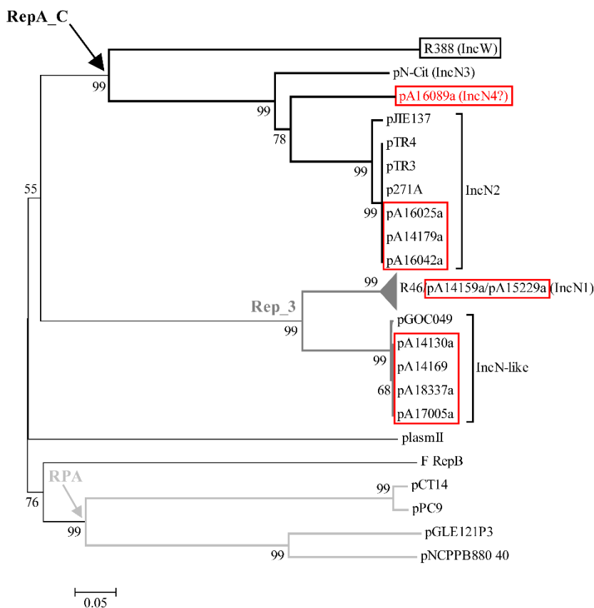
Figura 3.5.B. Filogenia de las proteínas iniciadoras de la replicación de los plásmidos MOB F11 /IncN secuenciados. Las proteínas iniciadoras de la replicación completas fueron alineadas utilizando AlignX y la filogenia se construyó mediante el programa Mega, tal como se ha explicado en la Sección 2. En las ramas de la misma está indicada la superfamilia Rep a la que pertenece cada una de las unidades taxonómicas representadas. Al final de las ramas, se indica el grupo de incompatibilidad de cada plásmido. El grupo IncN1 se encuentra comprimido por claridad La RepA del plásmido R388, modelo de la familia MOB F11 de relaxasas, aparece indicada por un recuadro gris claro. Las RepA de los plásmidos MOB F11 secuenciados y descritos en este apartado, aparecen indicados con un recuadro rojo. El plásmido pA16089a aparece con letras rojas para indicar que el grupo IncN4 es una suposición.
