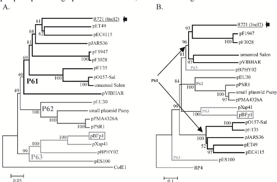
Figura 3.4.H. Filogenias de las proteínas relaxasa y VirB6/TraA de los plásmidos clasificados como MOB P6 . El panel A presenta la filogenia de las relaxasas MOBP6. Las proteínas incluidas en ella fueron obtenidas mediante el proceso ya explicado en la Sección 2. La filogenia fue reconstruída con los primeros 300 aminoácidos de cada una y siguiendo el método ya explicado en la misma sección. El panel B presenta la filogenia de la proteína TraH/TraA (homóloga de VirB6) de cada uno de los plásmidos anteriores. En este caso, se utilizó la proteína completa y dos métodos de reconstrucción para comprobar la robustez de la topología del árbol obtenido ( neighbour joining y UPGMA; el segundo no mostrado). El plásmido R721, modelo del grupo IncI2 y del MOBP6, aparece subrayado e indicado por una flecha negra. El plásmido pBFp1 aparece recuadrado en gris claro. Las distintas divisiones que se pueden establecer en MOBP6 aparecen indicadas en los nodos correspondientes y en colores: P61, negro; P62, gris; P63, gris claro.
