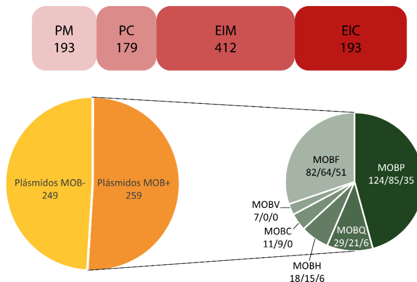
Figura 1.D. Diversidad y clasificación de los elementos móviles. En el panel superior se muestra la abundancia de los distintos elementos transmisibles por conjugación, encontrados en genomas procariotas completamente secuenciados (1207 cromosomas y 891 plásmidos, como se describe en [24]). PM indica plásmidos movilizables, PC indica los conjugativos, EIM indica los elementos integrativos movilizables y EIC los elementos integrativos conjugativos. En el panel inferior izquierdo se detalla la proporción de plásmidos transmisibles (MOB+) y no transmisibles (MOB-) encontrados entre los plásmidos de \gamma -Proteobacteria. En el panel inferior derecho se detalla la distribución de familias MOB entre los plásmidos de \gamma -Proteobacteria. Cada serie de números bajo la clase MOB indica, por este orden, el número de plásmidos en esta categoría, el número de ellos detectables por el método de clasificación de MOB por cebadores degenerados (DPMT) y el número de ellos detectables por PBRT, tal como se describe en [114]. Esta figura ha sido modificada de [14].
