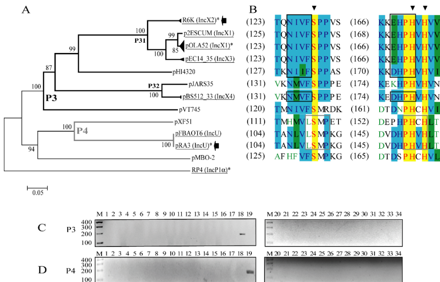
Figura 3.1.C. Validación del método DPMT para la familia MOB P3/P4 . A) Árbol filogenético de las relaxasas MOB P3/P4 . B) Alineamiento de los motivos de las relaxasas empleados en el diseño de las parejas de oligonucleótidos semi-degenerados ( P3-f+P3-r , negro continuo; P4-f+P4-r , gris oscuro continuo). C) Amplicones obtenidos con los oligonucleótidos correspondientes a la subfamilia MOB P3 ( P3-f+P3-r ). D) Amplicones obtenidos con los oligonucleótidos correspondientes a la subfamilia MOB P4 ( P4-f+P4-r ). Símbolos, colores y calles, igual que en la figura 3.1.A.
