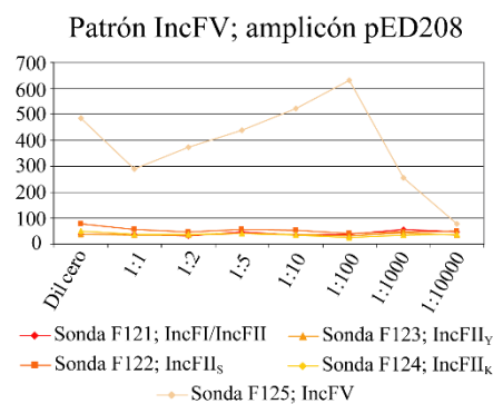
Figura suplementaria 3.2.B. Validación de las sondas MOB F12 para el array en suspensión. En el panel del patrón IncFII k , los valores U.F.A. iguales a cero corresponden a errores de lectura del hardware. Los ejes representan las mismas magnitudes que en el caso anterior.
