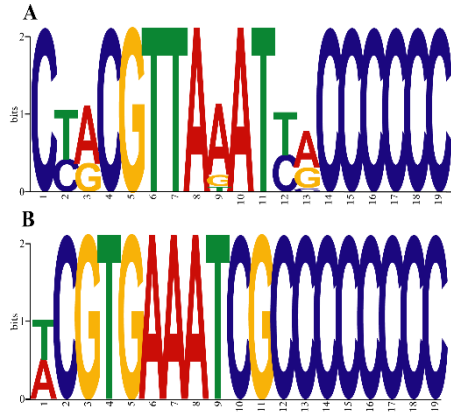
Figura 3.5.F. Logo del iterón consenso de los plásmidos MOB F112 /IncN2. Se predijeron, como ya se ha descrito, las secuencias y el número de iterones de los replicones de los plásmidos MOB F112 /IncN2 detallados en el texto. Presentamos la secuencia consenso de los mismos (panel A). Comparamos la secuencia de este iterón consenso con la del PAI MOB H2 pKLC102 (panel B). Las alturas de cada base responden a su frecuencia.
