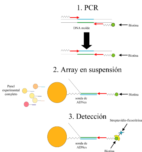
Figura 2.5.B. Flujo de trabajo del array en suspensión. Partimos de un amplicón producido con alguna de las parejas de oligos DPMT. Reamplificamos utilizando un oligo reverso modificado con biotina en 5' (flecha roja con esfera verde). El producto resultante se mezcla con el panel experimental utilizado, hibridándose con una de las secuencias diana en el mismo. A la mezcla se le añade estreptoavidina-ficoeritrina, que se une a la biotina, revelando su presencia. El láser detecta e identifica las microesferas por su emisión en el espectro del rojo, discriminando las rotas de las agregaciones múltiples y de los objetos individuales, que son los que contarán para el experimento. Otro láser detecta las microesferas que tienen una molécula de ADNcs hibridada a la correspondiente sonda, por medio de la emisión de la estreptoavidín-ficoeritrina en la longitud de onda del verde. La identidad del amplicón vendrá determinada por la identidad de la sonda asociada a la microesfera con la que hibridó la diana amplificada.
