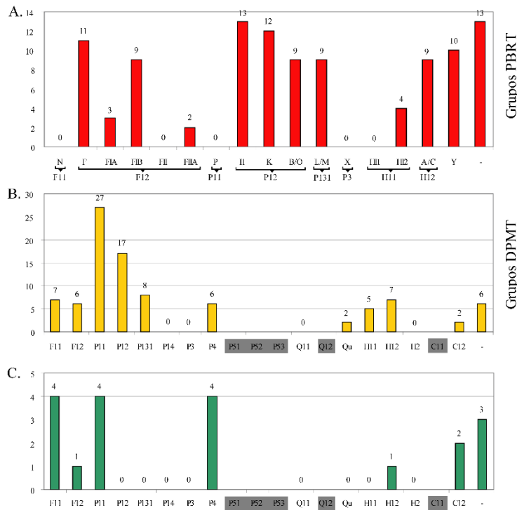
Figura 3.3.E. Caracterización de las cepas del Hospital Sant Pau i la Santa Creu por PBRT y DPMT. Comparación de los resultados obtenidos por los dos métodos en la misma colección de aislados. Cada categoría del eje de abscisas representa una pareja de cebadores de cada uno de los dos métodos. La gráfica A. detalla los resultados obtenidos con el método PBRT; bajo las categorías de cebadores PBRT se indica qué cebadores DPMT amplifica esta clase de relaxasas. La gráfica B. detalla los resultados obtenidos con el método DPMT. La gráfica C. indica los resultados del método DPMT sobre los aislados PBRT negativos. En todos los casos, el número de amplicones obtenidos se indica sobre cada barra. La última barra de cada gráfica indica el número de aislados inclasificables en cada uno de los dos métodos. Obsérvese que DPMT deja sin clasificar la mitad de aislados de los que deja PBRT. Las categorías sombreadas en gris en el eje de abscisas indican los cebadores DPMT no disponibles para esta colección. Para más detalles sobre cada aislado, véase la tabla suplementaria 3.
