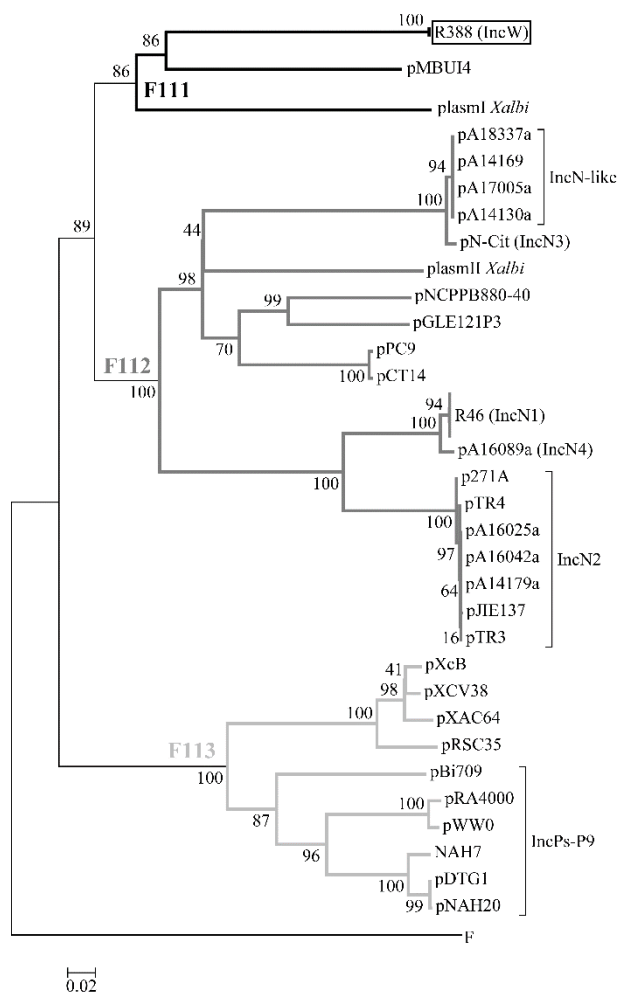
Figura 3.5.A. Filogenia de la subfamilia MOB F11 actualizada. La filogenia fue reconstruida de acuerdo a lo expuesto en la Sección 2, utilizando solo las relaxasas MOB F11 obtenidas en la iteración de convergencia. La filogenia está actualizada a fecha de Julio de 2013. La relaxasa TrwC de R388, modelo de la familia MOB F11 , aparece recuadrada. La nomenclatura de las ramas de la filogenia representa grupos de relaxasas sostenidos por valores de nodos estadísticamente significativos (esto es, >95) y es acorde con lo publicado anteriormente en [1-4]. Las ramas más importantes se muestran en colores distintos: F111 (negro), F112 (gris) y F113 (gris claro). Los grupos de incompatibilidad se indican en función de los datos bibliográficos o proporcionados empíricos (en el caso de las relaxasas nuevas incorporadas a la filogenia). pMBUI4 no está disponible en las bases de datos y se incorpora en esta filogenia por la amabilidad de la Dra. Eva Top. Xalbi se refiere a Xanthomonas albilineans , huésped de los plásmidos plasmI y plasmII.
