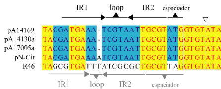
Figura 3.5.J. Alineamiento de los probables puntos de corte del oriT y las secuencias asociadas a una posible estructura secundaria. Se representan las secuencias de los tres plásmidos IncN-like de los que hablamos en el texto, comparándolas con las de los modelos IncN3 (pN-Cit) e IncN1 (R46). Los componentes del oriT de los plásmidos IncN3 e IncN4 están señalados en negro, mientras que los de R46 lo están en gris. El recuadro gris claro señala la secuencia conservada que contiene el probable sitio de corte. Éste está señalado igual que en la figura 3.5.D.
