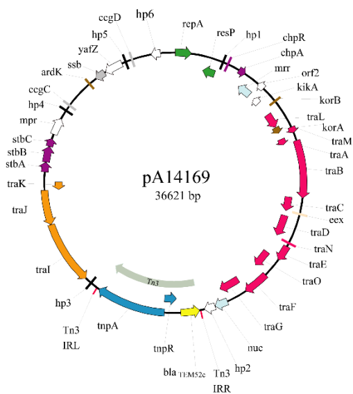
Figura 3.5.I. Mapa genético del plásmido pA14169. La leyenda de la figura es igual que la correspondiente de la figura 3.4.A.-
