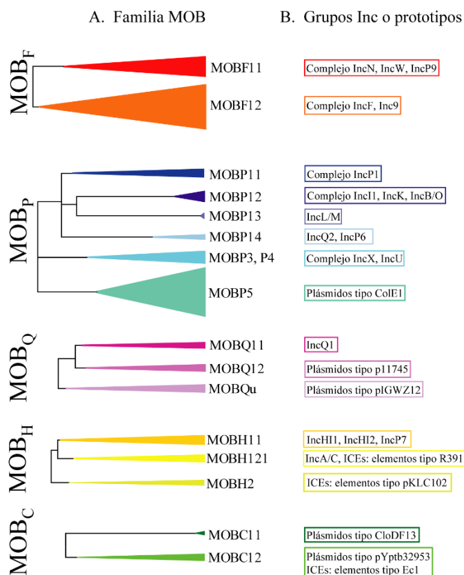
Figura 4.1.A. Correspondencia entre clases MOB y Inc/REP. A) Representación filogenética simplificada de las cinco familias MOB consideradas en el presente estudio. Los triángulos coloreados representan las subfamilias MOB amplificadas por DPMT. Su anchura y profundidad corresponden a la abundancia y diversidad de sus secuencias, respectivamente. B) Los grupos Inc/REP dentro de cada subfamilia MOB se indican en este panel, enmarcados bajo el mismo color. En ausencia de un grupo de replicación definido como grupo de incompatibilidad, se indica un plásmido prototipo.
