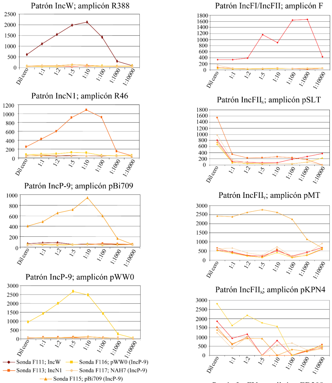
Figura suplementaria 3.2.A. Validación de las sondas MOB F11 para el array en suspensión. En los distintos paneles de esta figura se puede observar el comportamiento del panel experimental descrito en la leyenda de la misma, frente a distintos amplicones obtenidos como se describe en la sección 2.5. Sobre el eje de abscisas se representan las cantidades decrecientes de amplicón de doble cadena. Sobre el eje de ordenadas se representan unidades de fluorescencia arbitrarias (U.F.A.). cada punto representa la mediana de los valores de 100 mediciones individuales, como se explica en la sección 2.5. Las sondas F112 y F114 no se han añadido al panel experimental porque carecíamos de
