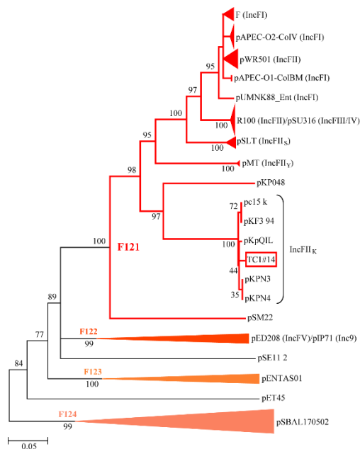
Figura 3.3.D. Filogenia de la subfamilia MOB F12 , actualizada con la relaxasa de TC1#14. Esta filogenia se ha reconstruido como ya se ha explicado (sección 2). Se ha evitado la rama de la subfamilia MOB F11 para aportar claridad a la figura. Del mismo modo, los otros cluster dentro de MOB F12 aparecen comprimidos, aunque se aportan ejemplos de plásmidos representativos para todos los casos. La nueva relaxasa aparece recuadrada en rojo. Para más información sobre esta familia MOB, acudir a la figura 3.1.A. y a su correspondiente texto asociado.
