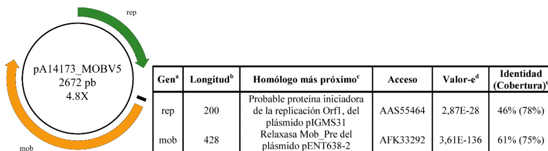
Figura 3.4.D. Mapa genético del plásmido pA14173_MOBV5 y tabla de los homólogos más próximos de sus productos protéicos. A la izquierda; el rectángulo negro indica la posición del oriT . El resto de colores y figuras, igual que en la figura 3.4.A. A la derecha:
