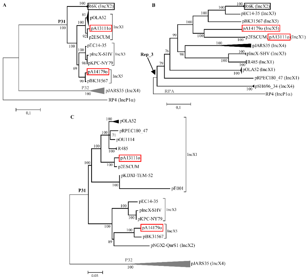
Figura 3.5.H. Filogenia de los plásmidos del complejo de replicación X. Las tres filogenias mostradas fueron construidas por medio de Mega4, tal como se ha explicado anteriormente (Sección 2.3.). El árbol A se obtuvo a partir de los 300 primeros aminoácidos de las relaxasas del grupo de replicación. El árbol B está construido a partir de la secuencia completa de la proteína iniciadora de la replicación de cada plásmido IncX, Pir. Por último, el árbol C está construido en base a las secuencias contiguas de las proteínas del chasis genético de los plásmidos IncX, tal y como se define en [13]. En todos los árboles, menos en el C , el plásmido modelo del grupo MOB p3 /IncX, R6K, aparece recuadrado en negro (no está completamente secuenciado y por ello no aparece en el árbol B ). Los plásmidos IncX descritos en las secciones 3.4. y 3.5. aparecen recuadrados en rojo. Algunas ramas aparecen comprimidas por claridad de la figura. En cada árbol se indica la familia relaxasa a la que pertenece cada grupo filogenético (árboles A y C ), la superfamilia de cada proteína iniciadora de la replicación (árbol B ) y el subgrupo del complejo IncX al que pertenecen (todos ellos). Los paneles A y B indican que pA14179o pertenece alternativamente a los subgrupos X5 y X1, respectivamente. Sin embargo, el panel C apoya claramente la topología propuesta en el panel A , por lo que afirmamos que forma parte de la rama IncX5, representada hasta ahora por pBK31567 [292].
