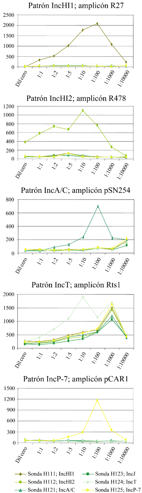
Figura suplementaria 3.2.I. Validación de las sondas MOB II para el array en suspensión. Las magnitudes son las mismas que en casos anteriores.
