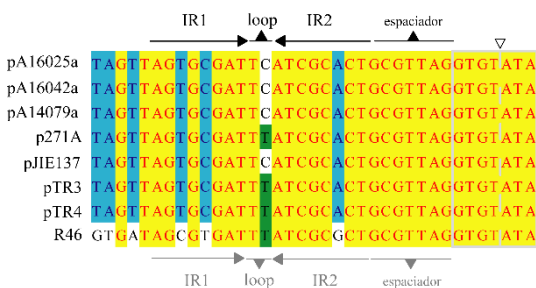
Figura 3.5.E. Alineamiento de los probables puntos de corte del oriT y las secuencias asociadas a una posible estructura secundaria. Se comparan las secuencias de los plásmidos IncN2 mencionados en el texto con la del modelo IncN1, R46. Los componentes del oriT de los plásmidos IncN2 están señalados en negro, mientras que los de R46 lo están en gris. El recuadro gris claro señala la secuencia conservada que contiene el probable sitio de corte. Éste está señalado por una cabeza de flecha blanca y una línea de puntos gris.
