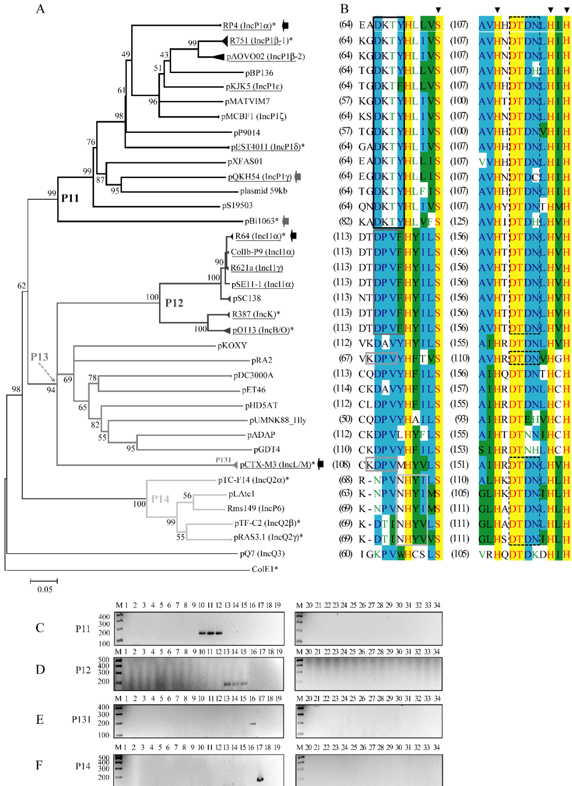
Figura 3.1.B. Validación del método DPMT para la familia MOB P1 . A) Árbol filogenético de las relaxasas MOB P1 . B) Alineamiento de los motivos de las relaxasas empleados en el diseño de las parejas de oligonucleótidos semi-degenerados ( P11-f , negro continuo; P12-f , gris oscuro continuo; P131-f , gris continuo; P14-f , gris claro continuo; P1-r , negro discontinuo). C) Amplicones obtenidos con los oligonucleótidos correspondientes a la subfamilia MOB P11 ( P11-f + P1-r ). D) Amplicones obtenidos con los oligos correspondientes a la subfamilia MOB P12 ( P12-f + P1-r ). E) Amplicones obtenidos con los oligos correspondientes a la subfamilia MOB P131 ( P131-f + P1-r ). F) Amplicones obtenidos con los oligos correspondientes a la subfamilia MOB P14 ( P14-f + P1-r ). Símbolos, colores y calles, igual que en la figura 3.1.A.
