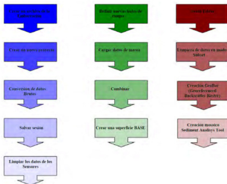
Figura 4.3. - Flujo de trabajo en el entorno de r s para el procesado de la reflectividad obtenida con ecosonda multihaz.
