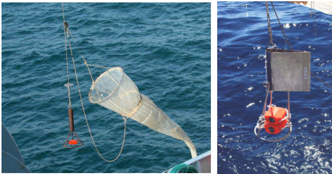
Figura 4.8.1. A) Detalle de la red WP2 y B) del sistema de posicionamiento basado en sensores Scanmar.
