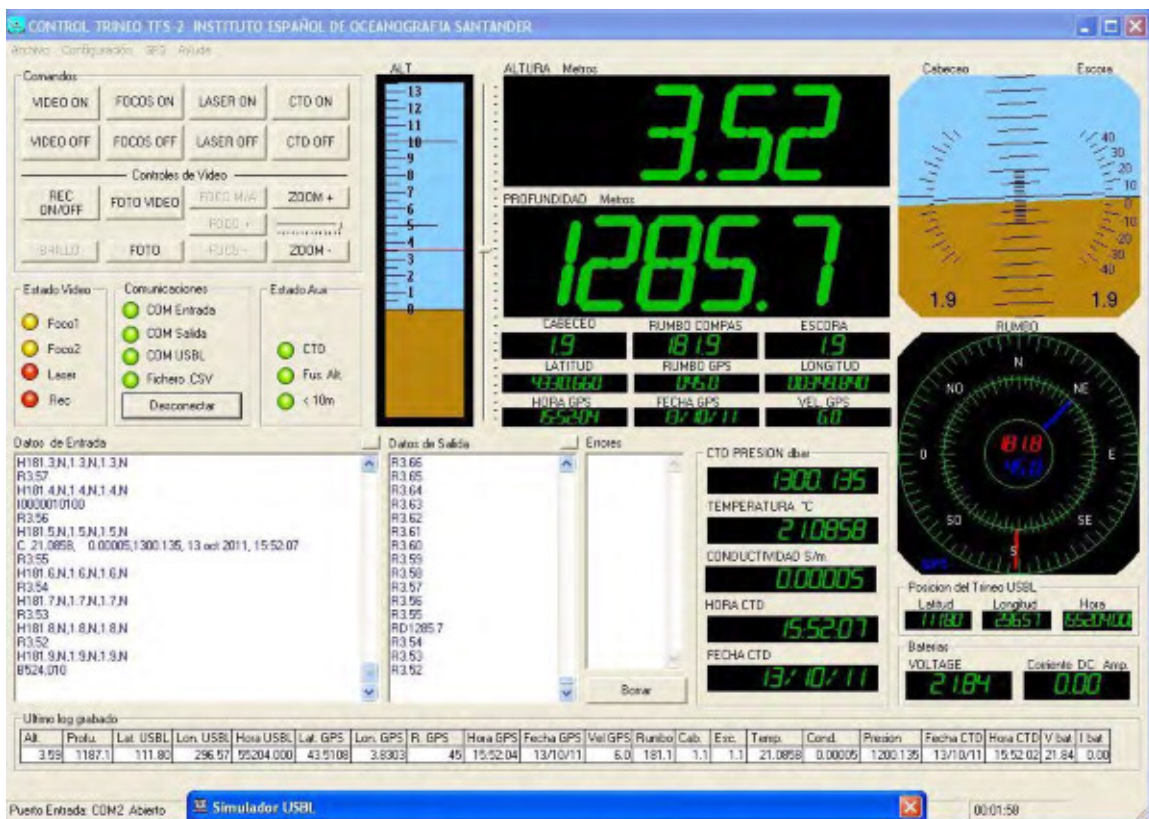
Figura 4.10.10. er ce del programa de control de vuelo (versión 2012) de los trineos y o o que integra y sincroniza la telemetría de los diferentes subsistemas para la monitorización de los transectos visuales directos con los vehículos submarinos. En la tabla inferior con encabezado “Ultimo log grabado” se muestran los parámetros archivados cada segundo.
