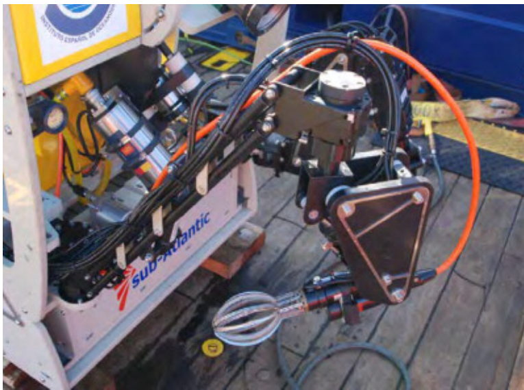
Figura 4.10.2.- A) Brazo manipulador de 6 grados de libertad ro e HLK-47000 (a la izquierda) para la captura de ejemplares vivos y B) sistema de succión acoplado al manipulador ro e HLK-HD45 de 5 funciones (a la derecha).
