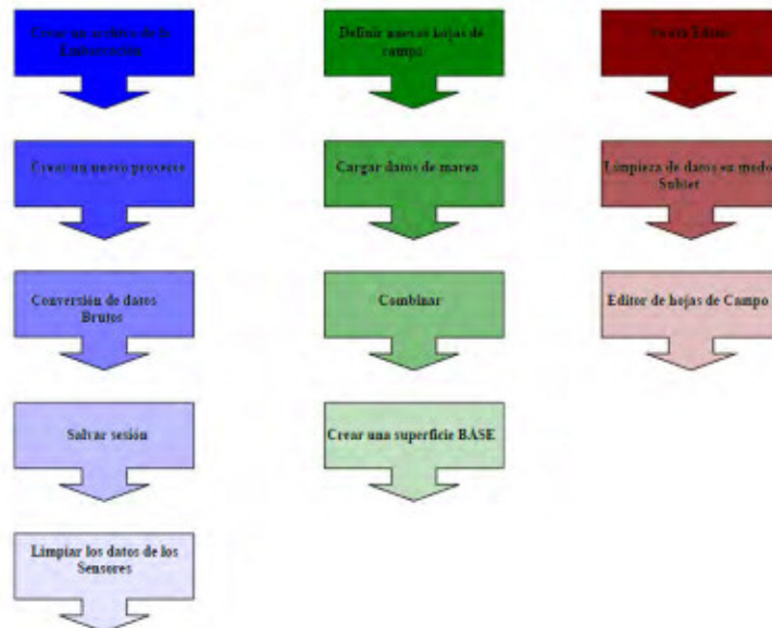
Figura 4.3.5.- Flujo de trabajo en el entorno de rs s para el procesado de las sondas obtenidas con ecosonda multihaz.
