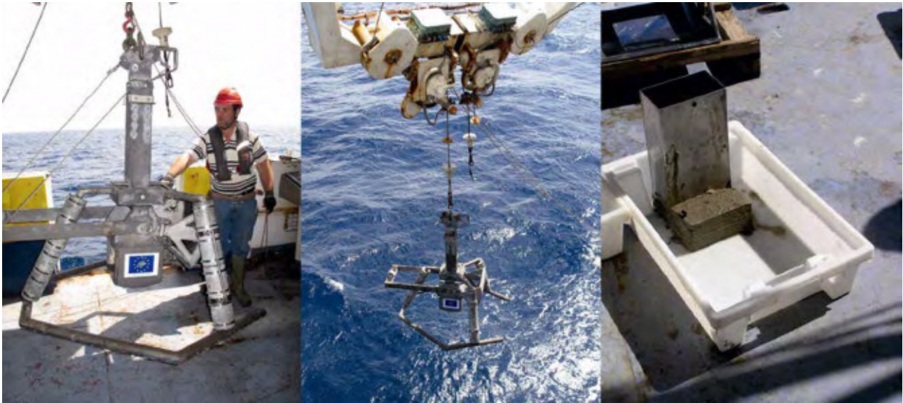
Figura 4.3.13.- Draga mesobox corer a bordo, recuperación de la draga y preparación de muestras.
