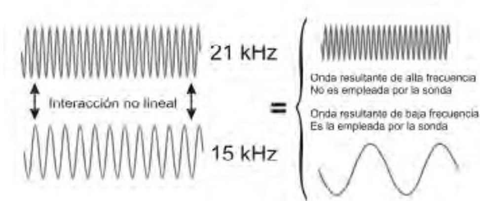
Figura 4.3.11- Esquema ilustrativo de la generación del efecto paramétrico.
