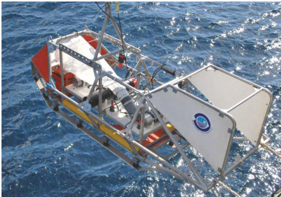
Figura 4.10.6.- Trineo fotogramétrico durante la campaña A0912. Se puede observar la disposición de la red para la captura de organismos suprabentónicos sobre hábitats de fondos duros tridimensionalmente complejos.
