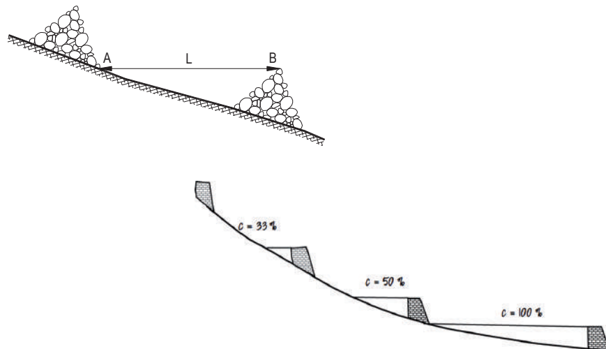
Figura 3.2.8.2. Diferentes estrategias de espaciado óptimo de diques de contención, siendo c=100\% la más segura y eficiente (de Gómez et al. 2019)
