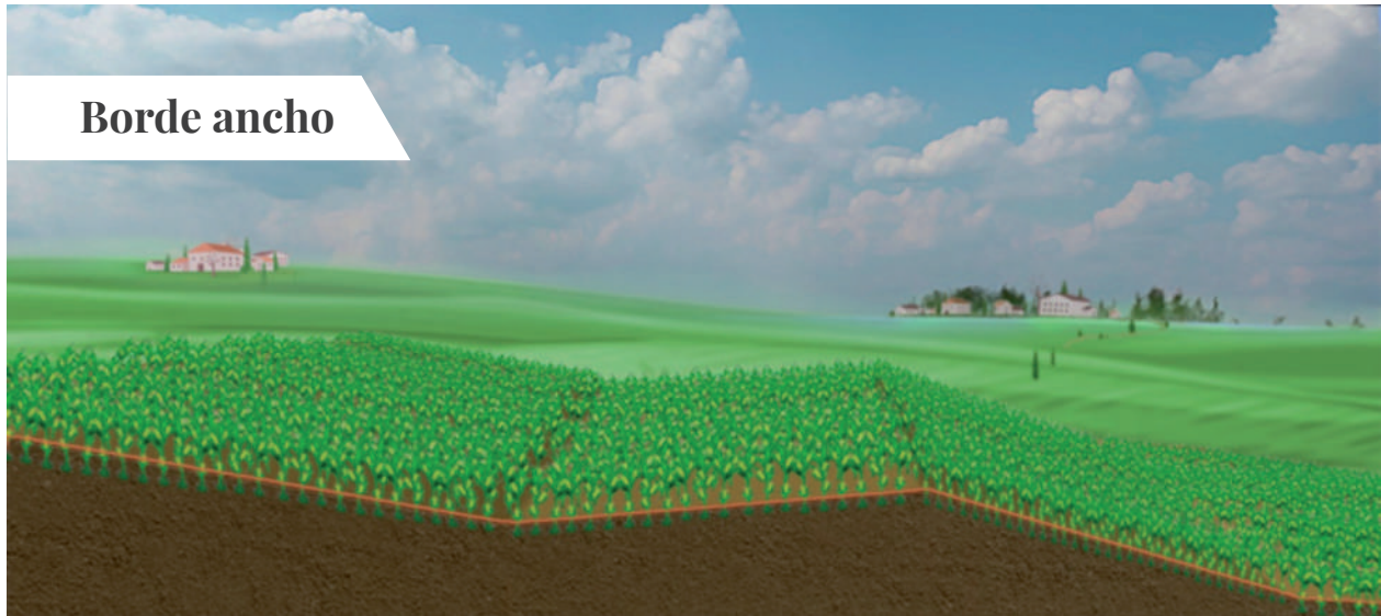
Figura 3.2.1.3a. Comparación de terrazas según su sección transversal: Borde ancho, borde estrecho y banal de conservación.
