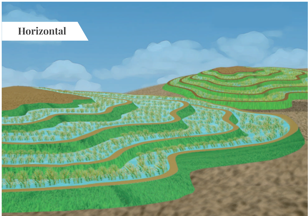
Figura 3.2.1.4. Comparación de terrazas según su clasificación: Horizontala vs. en pendiente.
