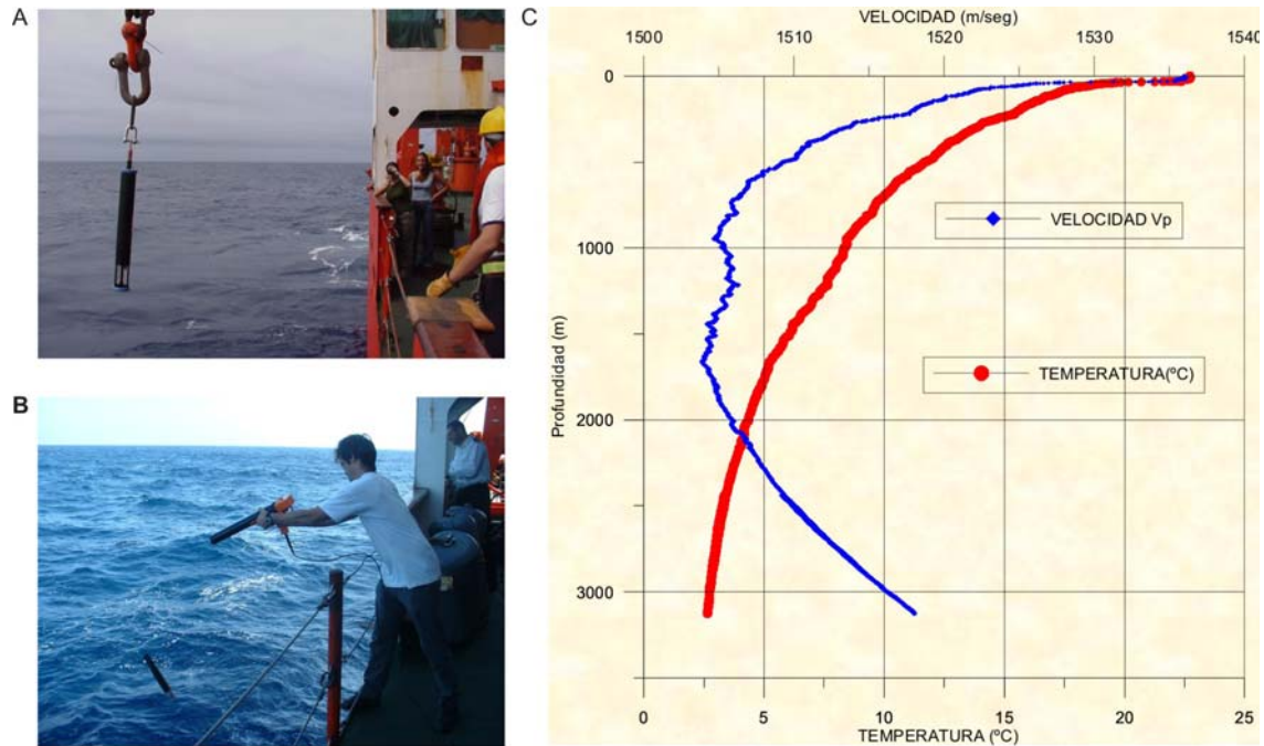
Figura 10.- Largado del sensor de la sonda SVplus. B. Lanzamiento de un batitermógrafo desechable (XBT). C. Curvas de velocidad de sonido y temperatura en la columna de agua.
