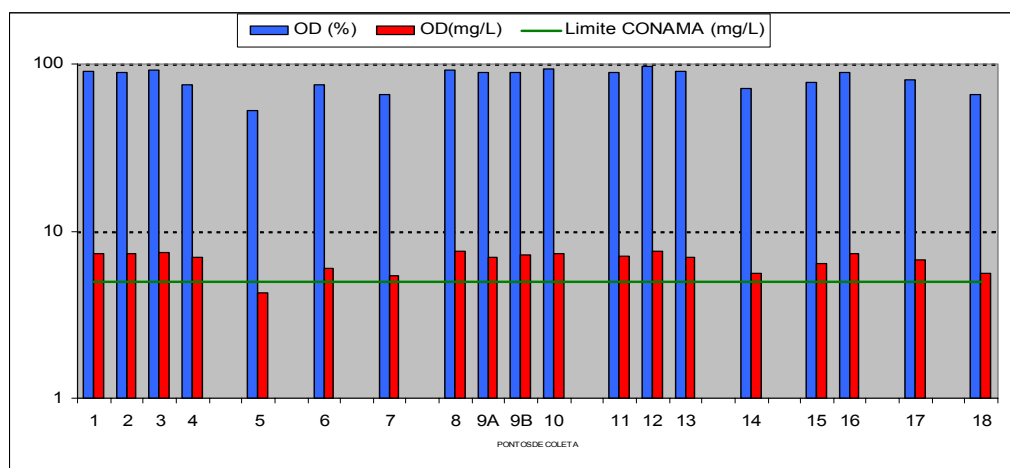
Figura 24. Oxigênio dissolvido medido em pontos selecionados de drenagens da área do PESCA e zona de influência e Limite Mínimo Permissível segundo Resolução nº 20/1986 do CONAMA.
