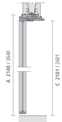
Slim Porta battente Swing door
