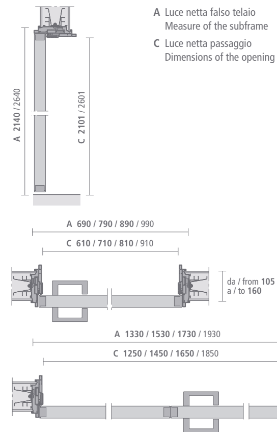
Slim Porta battente Swing door
