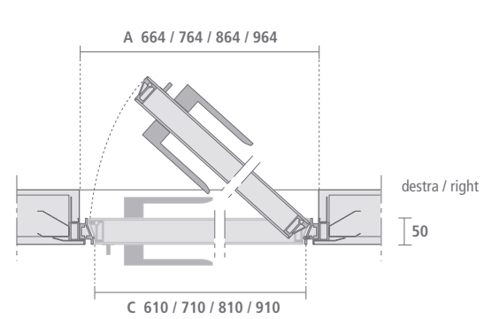
Porta con apertura a spingere Door with push opening
