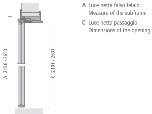
Porta battente Swing door
