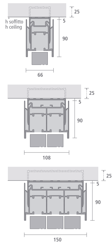
Binario a soffitto Ceiling rail
