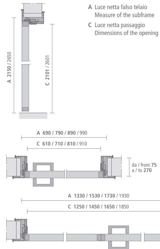
Porta battente Swing door
