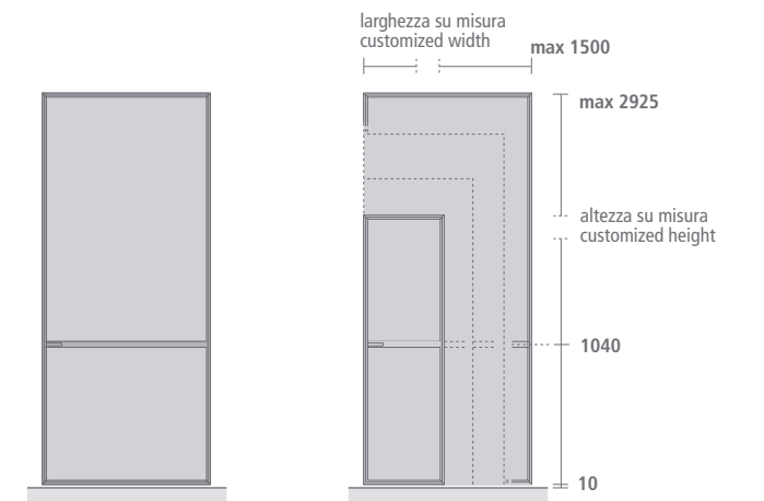
Pannello con traverso Cross panel
