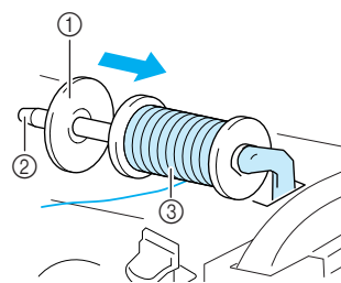
① Zusätzlicher Garnrollenstift ② Garnrollenkappe ③ Garnrolle
