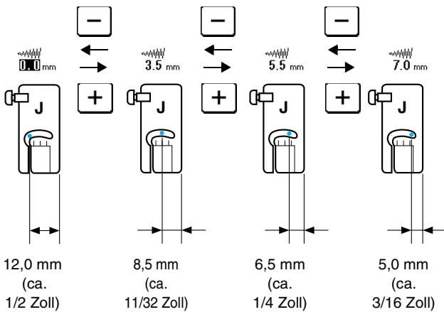
① Stichbreite
