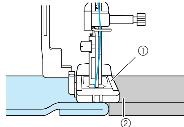
① Nähfuß ② Dicker Stoff
