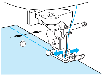
① Stichbreite
