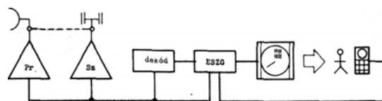
4. ábra: Automatizált repülésirányító munkahely rádiolokációs csoportosítása
