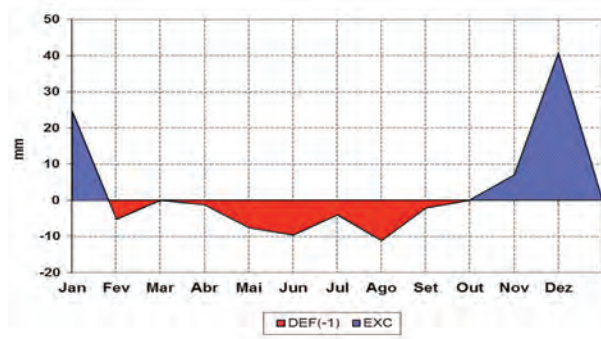
Figura 4: Balanço hídrico de Thornthwaite & Mather (1955) para Linhares/ES, de 1975 a 2004.
