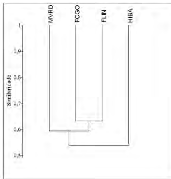
Figura 2: Dendrograma obtido por análise de agrupamento (UPGMA) a partir de listas florísticas de quatro regiões da Floresta Atlântica no leste do Brasil. Coeficiente de correlação cofenética = 0,61. FLIN, floresta de Linhares; HIBA, Hileia Baiana; MVRD, médio vale do rio Doce; FCGO, Falha de Campos dos Goytacazes.
