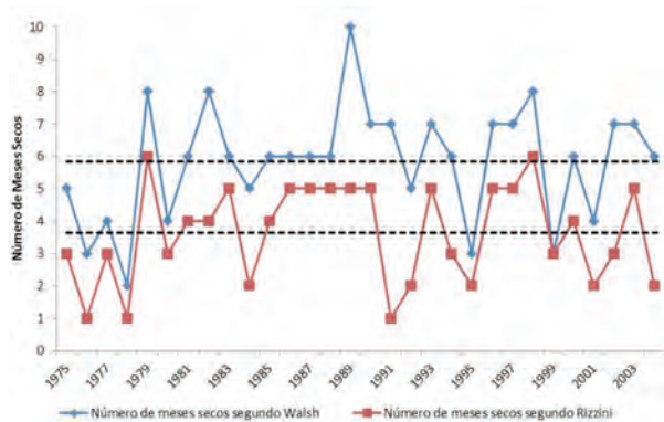
Figura 3: Frequência de meses secos entre os anos de 1975 e 2004 em Linhares/ES, de acordo com Walsh (1996b) e Rizzini (1997). O tracejado indica o número médio de meses secos em cada método.
