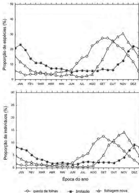
Figura 5: Variação anual média da intensidade da mudança foliar de árvores do dossel da Reserva de Linhares/ES. As proporções apresentadas referem-se à porcentagem média de ocorrência quinzenal de espécies (gráfico superior) e indivíduos (gráfico inferior) com as fenofases: árvore desfolhada (queda de folhas); brotação e copa constituída por folhagem totalmente nova (folhagem nova), no período de maio-82 a dezembro-92. Fonte: Engel, 2001.
