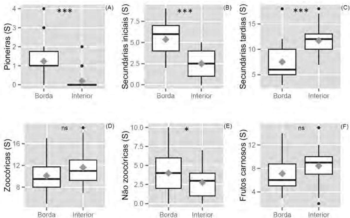
Figura 2: Comparação dos valores de riqueza de espécies por atributo funcional entre os habitats de borda e interior estudados nas Reserva Natural Vale e Rebio de Sooretama. (A) Pioneiras; (B) Secundárias iniciais; (C) Secundárias tardias; (D) Zoocóricas; (E) Não zoocóricas; (F) Frutos carnosos. * <0,05 ; ** <0,01 ; *** <0,001 ; ns=Não significativo; Diamantes cinza representam a média dos valores; Círculos pretos representam possíveis outliers.
