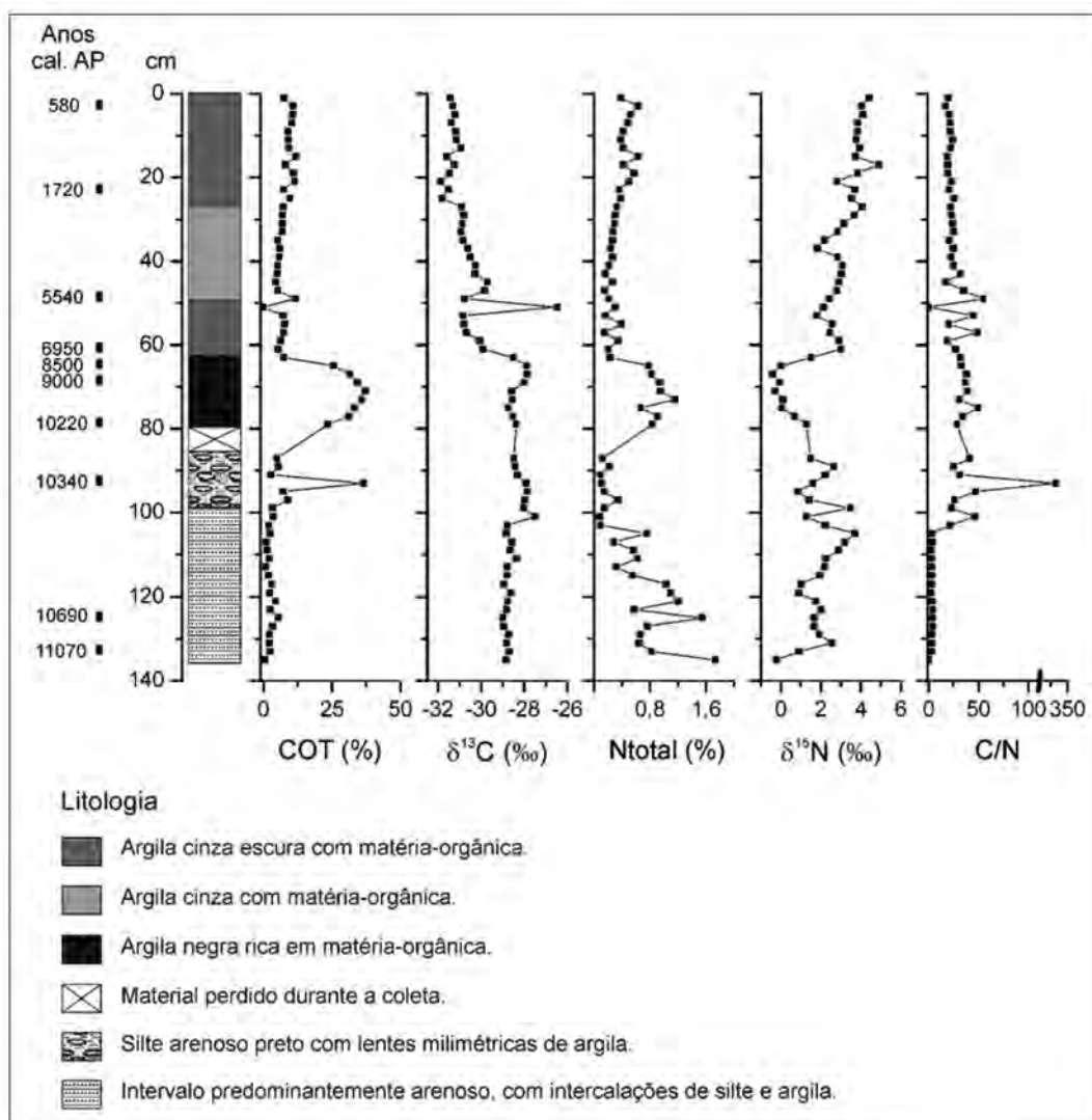
Figura 3: Análises isotópicas e elementares de C e N no testemunho LCGB.
