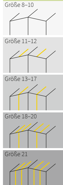
Gestängeskizzen - Serienausstattung - empfohlene Zusatzstangen (siehe S. 79)
