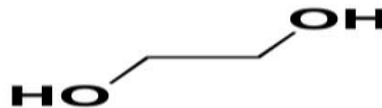
1,2-ethanediol (ethylene glycol)
