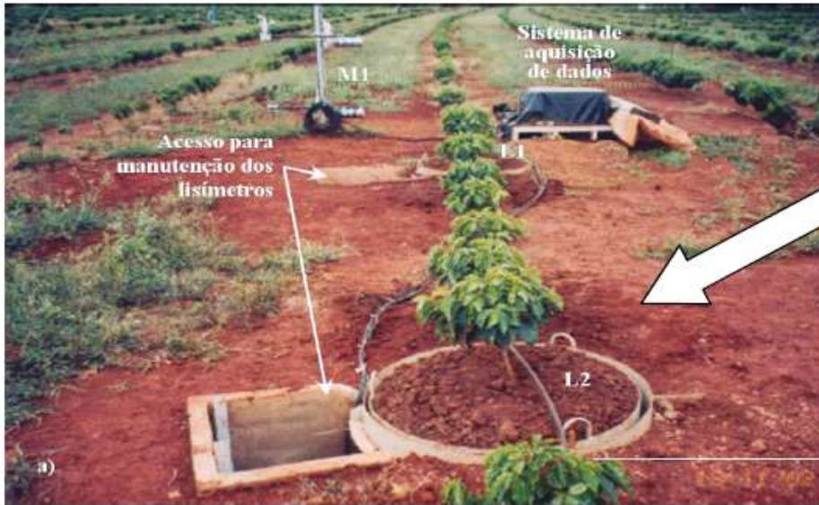
Lisímetro de pesagem para a medida da ET do cafeeiro
