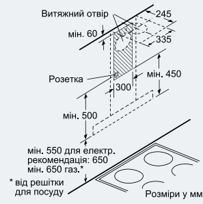
Розміри у мм
