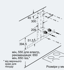
Розміри у мм
