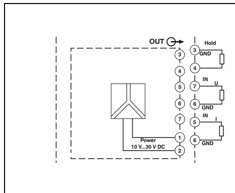
Blockschaltbild MCR-SL-D-SPA-UI
