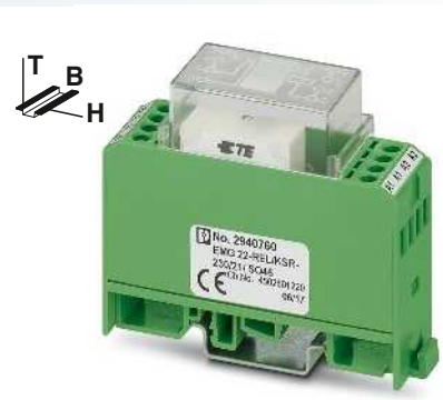
1-Wechsler, eingelötetes Relais
