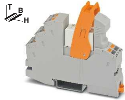
1-Schließer-Relaismodul mit Push-in- und Schraubanschluss
