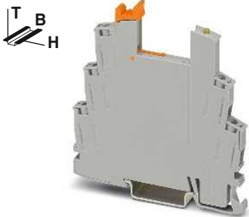
1-Wechsler-Relaissockel mit Schraubanschluss-technik
