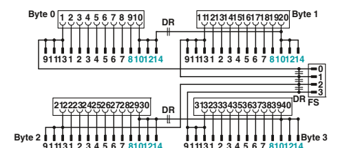
Anschlussbild FLKM 50/4-FLK14/PA-S300
