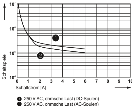
Elektrische Lebensdauer für PLC-R.../21HC...
