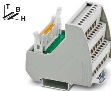
26- bis 64-polig mit Schraubanschluss
