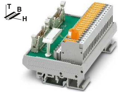
Passives Übergabemodul für SIMATIC® S7-300 mit Messertrennklemmen
