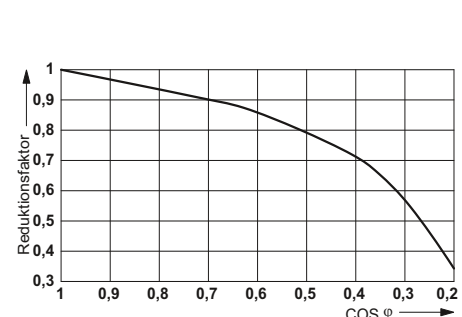
Lebensdauer-Reduktionsfaktor
