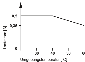
Derating-Kurve für PLC...24DC/48DC/500/W
