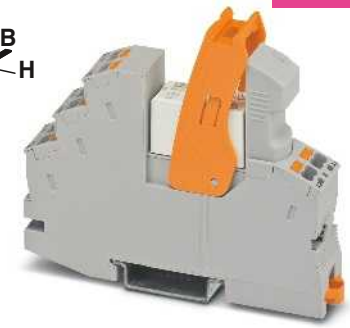
1-Schließer-Relaismodul mit Push-in- und Schraubanschluss
