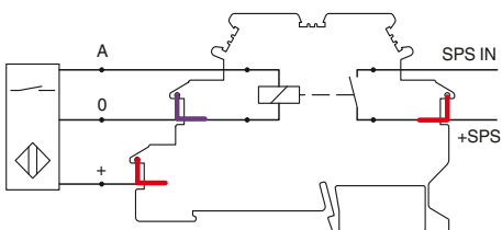
Anschlussbelegung DEK-REL-...SEN
