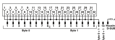
Anschlussbild FLKM-PA-2D15/HW/DI/C300
