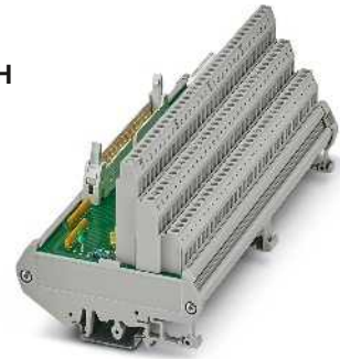
Initiatormodule für 32 Kanäle, mit Schraubanschluss und Leuchtanzeige
