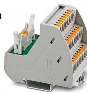
Initiatormodule für 8 Kanäle mit Push-in-Anschluss
