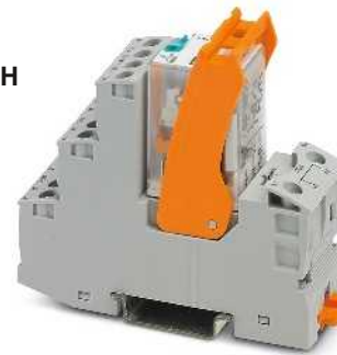
2-Wechsler-Industrirelaismodul mit Schraubanschluss und Handbetätigung
