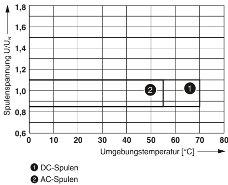
Betriebsspannungsbereich
