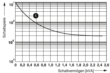
Elektrische Lebensdauer
