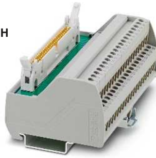
Passives Übergabemodul für Modicon® TSX Quantum™ mit Schraubanschluss
