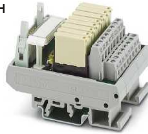
Ausgabemodul mit 8 Miniaturrelais, 1 Schließer
