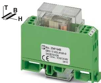
für mittlere bis große Leistungen 1 Schließer (1)
