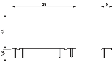
5 mm Baubreite
