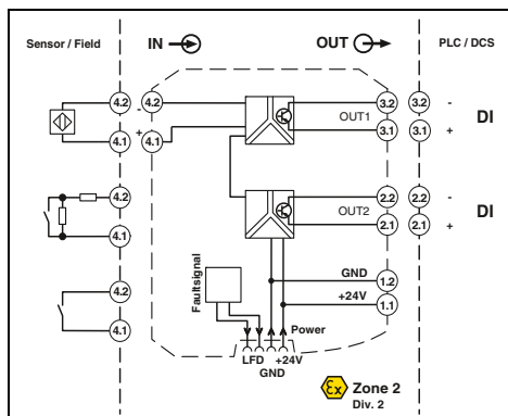
NAMUR-Trennschaltverstärker, 2 Signalausgänge: Transistor (passiv)
