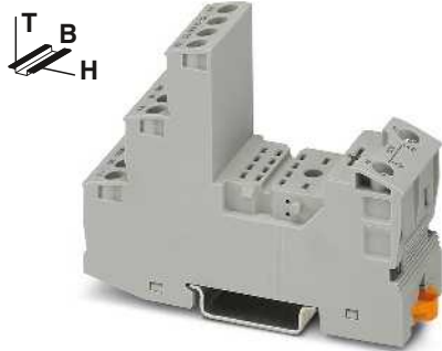
4-Wechsler-Relaissockel mit Schraubanschlusstechnik für Industrirelais
