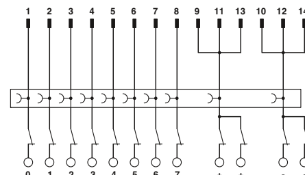
Anschlussbild FLKM 14/KDS3-MT/PPA/PLC
