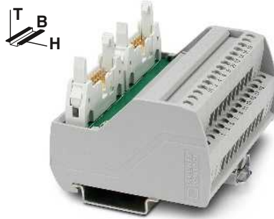
Passives Übergabemodul für Allen Bradley ControlLogix mit Schraubanschluss
