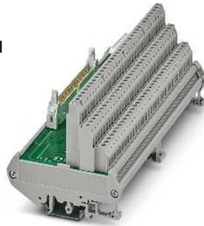
Initiatormodule für 32 Kanäle, mit Schraubanschluss
