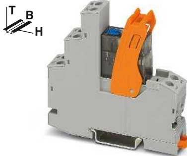
2-Wechsler-Relaismodul mit Schraubanschluss und Handbetätigung
