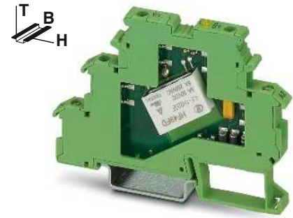
für kleine bis mittlere Leistungen 1 Schließer (1)
