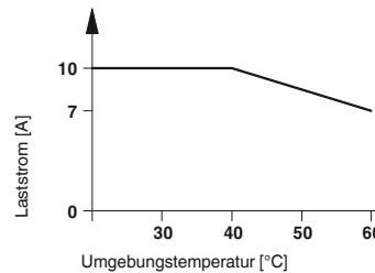
Derating-Kurve für PLC...24DC/24DC/10/R
