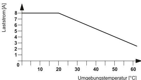
Laststrom in Abhängigkeit von der Umgebungstemperatur Einschaltdauer: 100% ED
