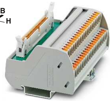
Passive Übergabemodule für Ein-/Ausgabe mit Push-in-Anschluss
