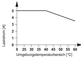
Derating-Kurve für Solid-State-Relais OPT...DC/230AC/2 und PLC-OS.../230AC/2/ACT
