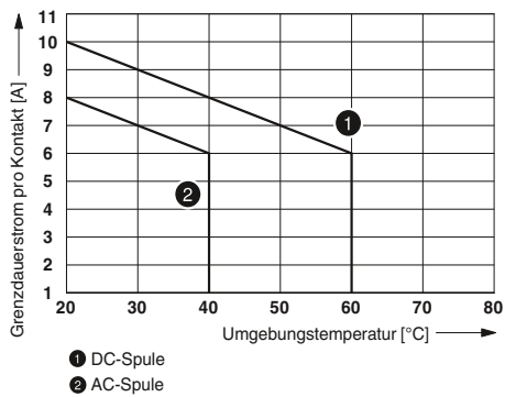
Kontaktderating
