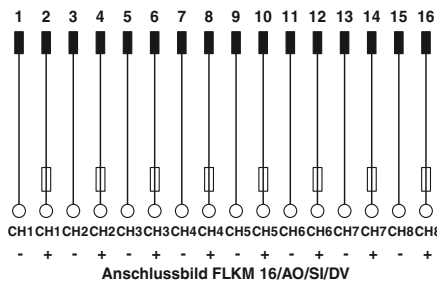
Anschlussbild FLKM 16/AO/SI/DV
