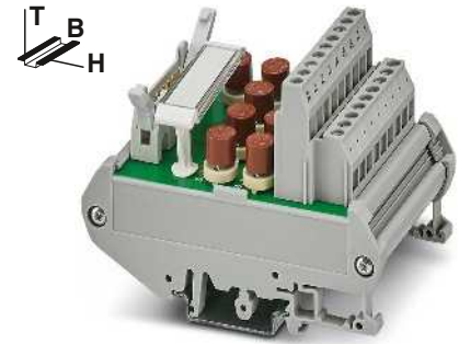
Passive Sicherungsmodul für 8 bzw. 32 Kanäle
