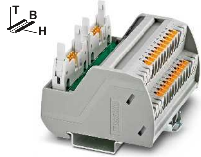
Passives Übergabemodul für Allen Bradley ControlLogix mit Push-in-Anschluss
