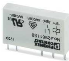
Relais mit einem Wechslerkontakt, max. 6 A
