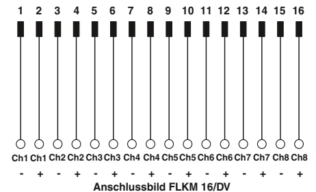
Anschlussbild FLKM 16/DV
