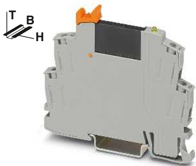
Solid-State-Relaismodul mit Schraubanschluss, DC-Ausgang max. 100 mA
