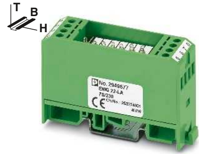
Leuchtanzeigemodul, mit gemeinsamer Rückleitung
