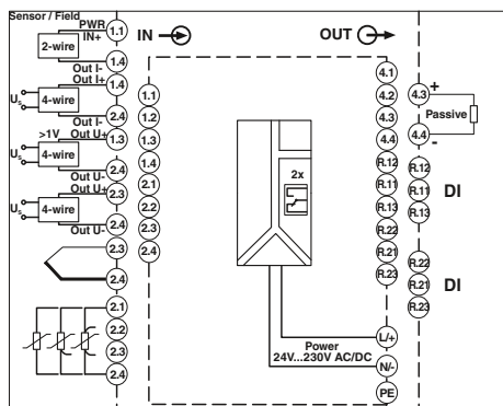
Blockschaltbild FA-MCR-D-TUI-UI-2REL-UP
