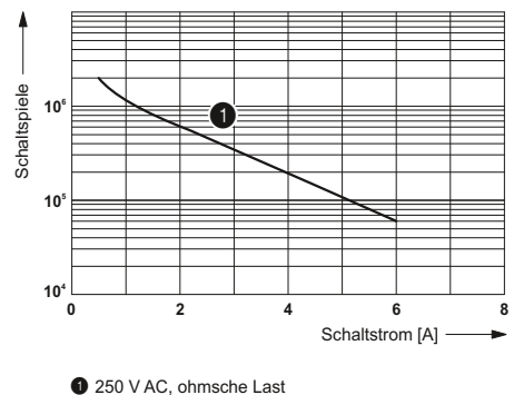
Elektrische Lebensdauer
