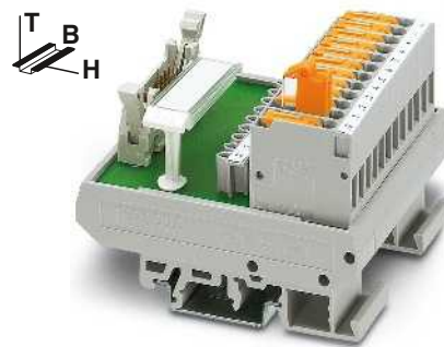
Passive Übergabemodule für 8 bzw. 32 Kanäle mit Messertrennklemmen
