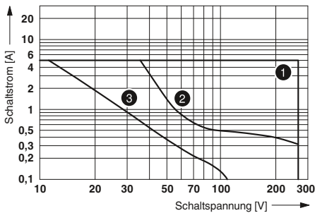
Abschaltleistung
