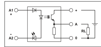
Bild 4: Der 3-Leiterausgang
