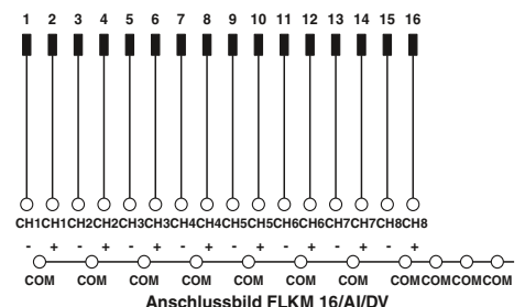
Anschlussbild FLKM 16/AI/DV
