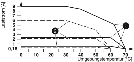
Derating-Kurve für ELR H3...230AC...
