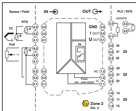
Temperaturmessumformer, universell, mit drei Grenzwert-Relais, Weitbereichsversorgung
