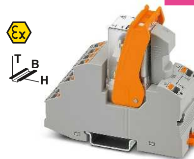
4-Wechsler-Industrirelaismodul mit IECEx-, ATEX- und Cl. 1 Div. 2-Zulassung
