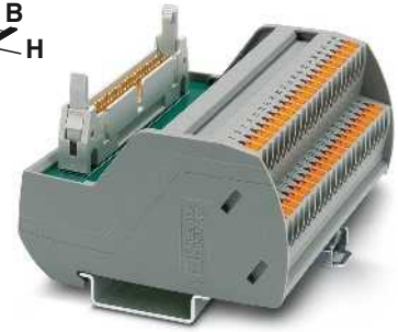
Passive Übergabemodule für SIMATIC® S7-400 mit Push-in-Anschluss
