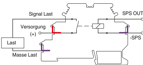
Anschlussbelegung DEK-REL-...AKT
