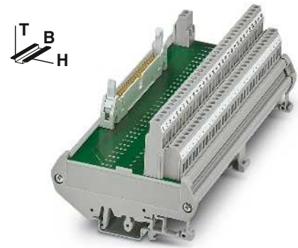
Übergabemodule für DeltaV mit 2-Leiter-Schraubanschluss
