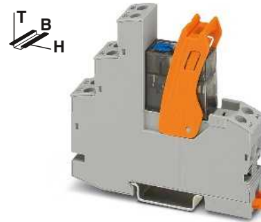
1-Wechsler-Relaismodul mit Schraubanschluss und Handbetätigung
