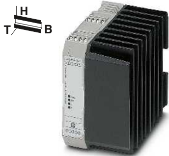
zum Reversieren von 3~ AC-Motoren bis 575 V AC/3 x 9 A
