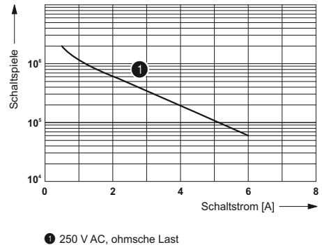
Elektrische Lebensdauer
