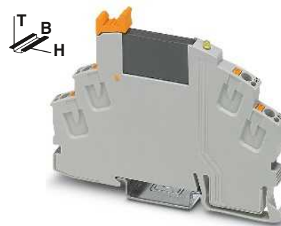
Solid-State-Relaismodul mit Push-in-Anschluss, DC-Ausgang max. 3 A
