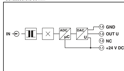
für Gleich-, Wechsel- und verzerrte Ströme 0...300 A, Spannungsausgang
