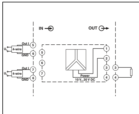
Blockschaltbild MCR-SL-S-U-I
