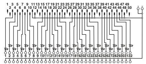
Anschlussbild FLKM 50/32M/IN/LA/DV
