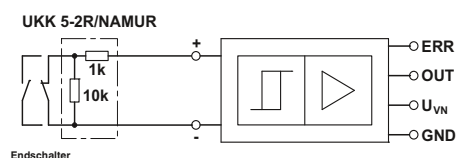
Applikation 2
