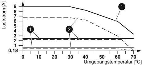
Derating-Kurve für ELR H3...24DC...
