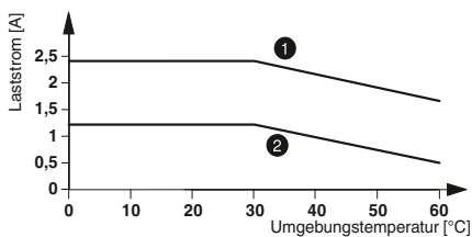
Laststrom in Abhängigkeit von der Umgebungstemperatur Einschaltdauer: 100% ED
