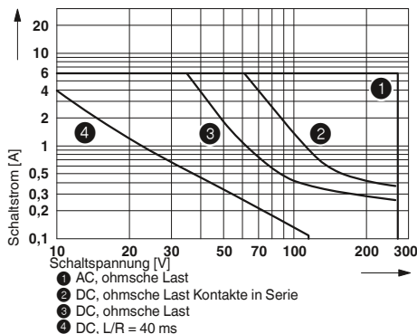
Elektrische Abschaltleistung für PLC...1IC/ACT für hohe Einschaltströme
