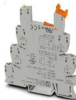
1-Schließer-Grundklemme zur Bestückung mit Relais für TTL (5 V)
