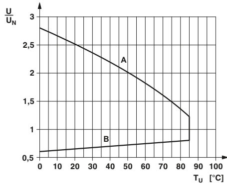
Eingangsspannungsbereich
