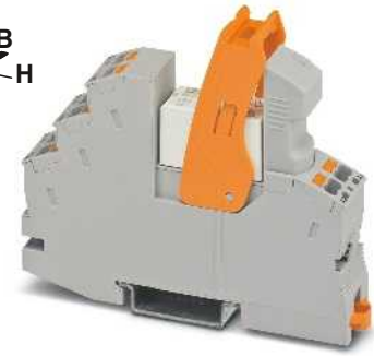
1-Wechsler-Relaismodul mit Push-in-Anschluss
