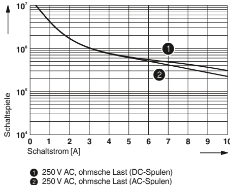
Elektrische Lebensdauer für PLC-R.../21HC...
