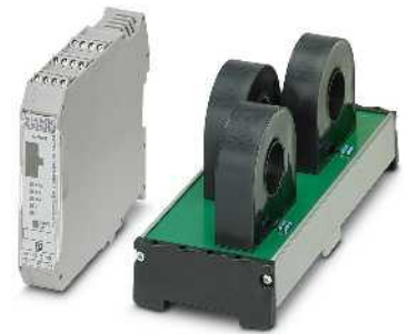
mit externen Stromwandlern bis 160 A
