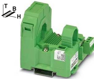
für sinus- und nicht sinusförmige Wechselströme 0...200 A, Spannungsausgang
