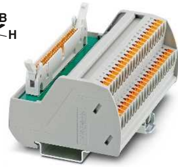
Passives Übergabemodul für Modicon® TSX Quantum™ mit Push-in-Anschluss
