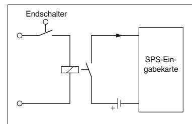
Applikationsbeispiel: SPS-Eingabesignal
