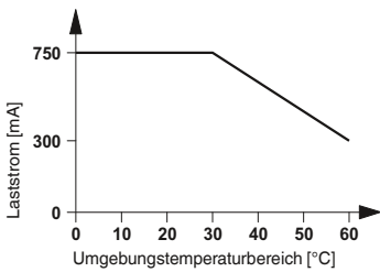
Derating-Kurve für Solid-State-Relais OPT...DC/230AC/1 und PLC-OS.../230AC/1
