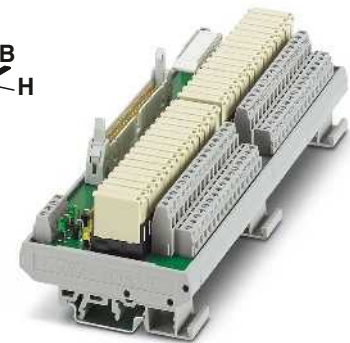
Ausgabemodul mit 32 Miniaturrelais, 1 Schließer
