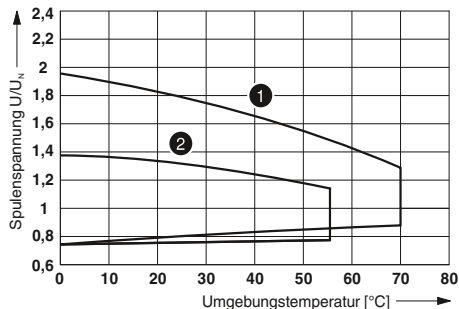
Betriebsspannungsbereich
