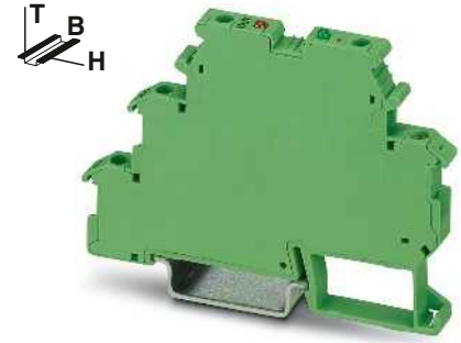
für induktive Näherungsinitiatoren nach NAMUR
