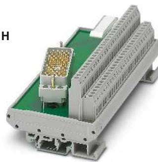
56-polig
