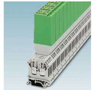
Leistungs-Solid-State-Relais mit 400 V AC / 3 A-Ausgang
