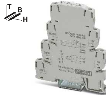
Zeitrelais mit Blinkerfunktion, impulsbeginnend
