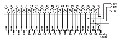
Anschlussbild FLKM-PA-D37/ETHA
