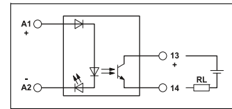
Bild 3: Der 2-Leiterausgang
