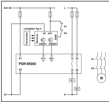
PSR-MS60 – Zweikanalige Lichtgitterüberwachung mit automatischem Start
