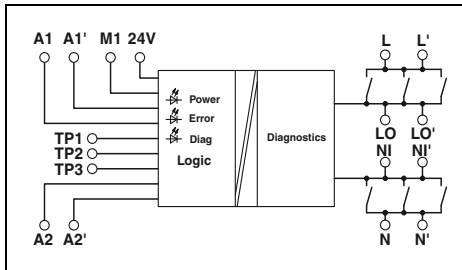
SIL-3-zertifiziertes Koppelrelais zum sicheren Einschalten (F&G), Off-State-Diagnose
