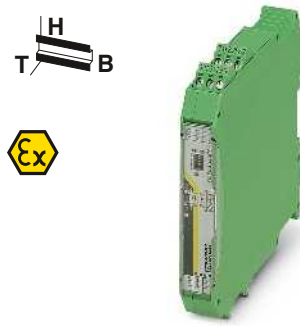
4 analoge Strom-/Spannungsausgänge
