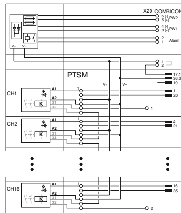
Anschlussbild TC-2D37SUB-DO16-ESD-AR-UNI
