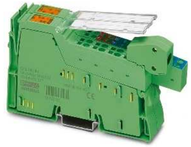
Eingang für Inkremental-Encoder mit Rechtecksignal (symmetrisch oder asymmetrisch)
