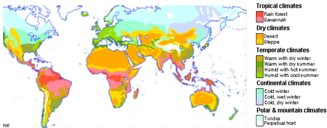
Fig 4. World climate zones (Köppen-system)
