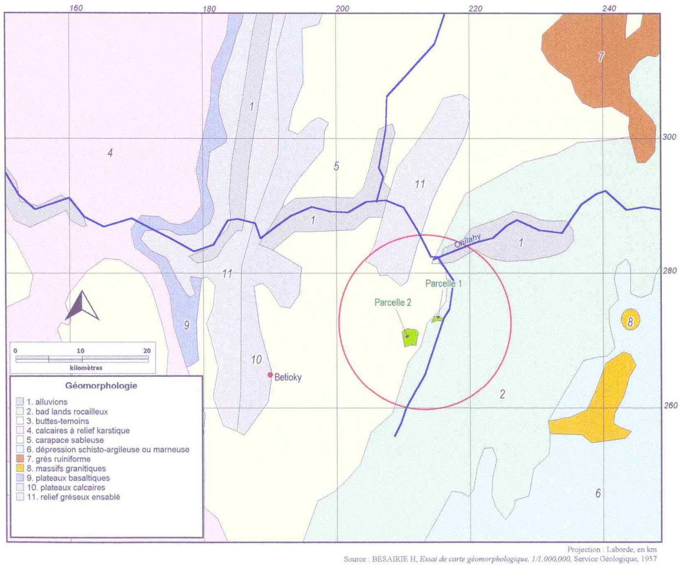
Carte 3 : Géomorphologie de la région de Beza Mahafaly
