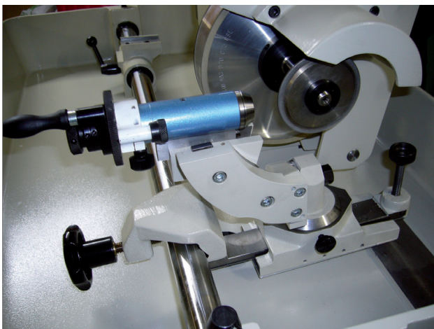
Nr. 6.22 Universal Schleifapparat Universal grinder
