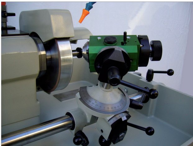
Nr. 6.20 Bohrer- und Fräuserschleifapparat Drill- and milling cutter grinder
