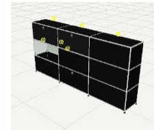
Sideboard USM Haller Design: Fritz Haller B/T/H: 225/35/109 cm Abdecktablare mit Resopal 0901 beschichtet, mit 4 Klapptüren (1 x mit Schloss) 1 HR Auszug und 3 offenen Fächern davon 1 x mit Beleuchtung und verspiegelten Seiten- und Rücktablar (Sonderanfertigung- Preis auf Anfrage)
