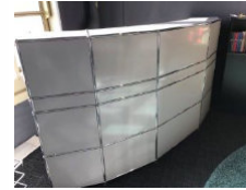
Rundtheke USM ** Auslaufmodell - nicht nachbestellbar ** Maße B/T/H 242/65/119 cm Ausführung: Rückseite & Außenseiten geschlossen 5. Reihen mit Aufteilung in 4x Elemente: 4. Reihen beinhalten 3x USM- Tablare/Böden
