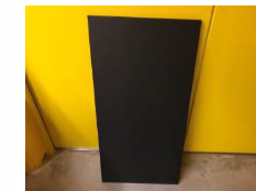
Abdeckplatte für Standcontainer VersaS Maße: B/T 44,3 x 90 cm Zum Aufstecken mittels M1- Stiften, jeweils 5 mm Schattenfuge als Aufdopplung 5 mm MDF schwarz, links, rechts & hinten 5 mm eingerückt, Plattendicke: 19 mm E1, Oberfläche: "H6" Soft Touch, Farbe: schwarz
