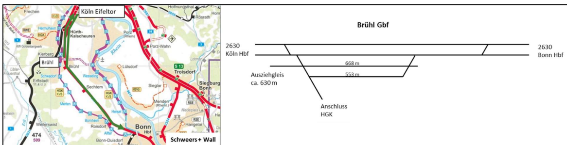
Abbildung 9: Fahrten von und nach Brühl Gbf verkehren über Köln Eifelort und der Gleisplan von Brühl Gbf
