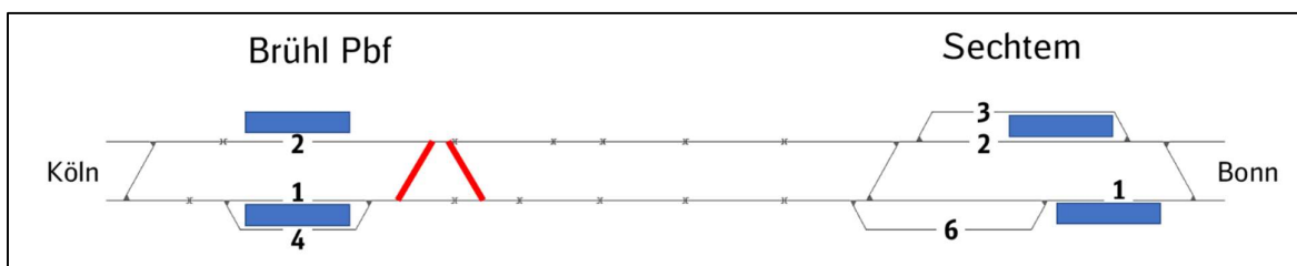
Abbildung 18: Zwei zusätzliche Weichen zwischen Brühl und Sechtem
