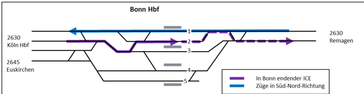
Abbildung 11: Fahrwegüberschneidungen bei der Ausfahrt aus Gleis 2 in Richtung Süden in Bonn Hbf
