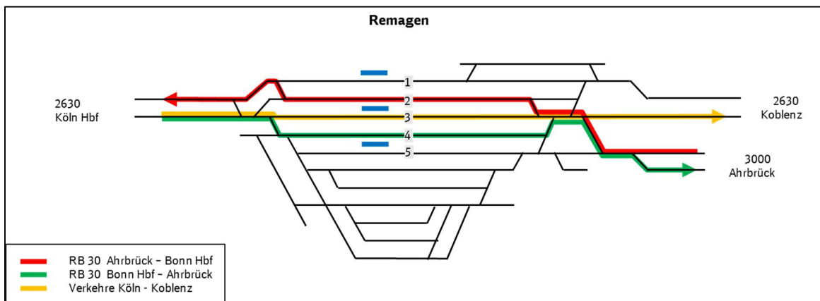
Abbildung 13: Fahrwegüberschneidungen in Remagen
