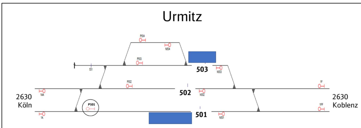
Abbildung 26: Zusätzliches Ausfahrtsignal P501 in Urmitz
