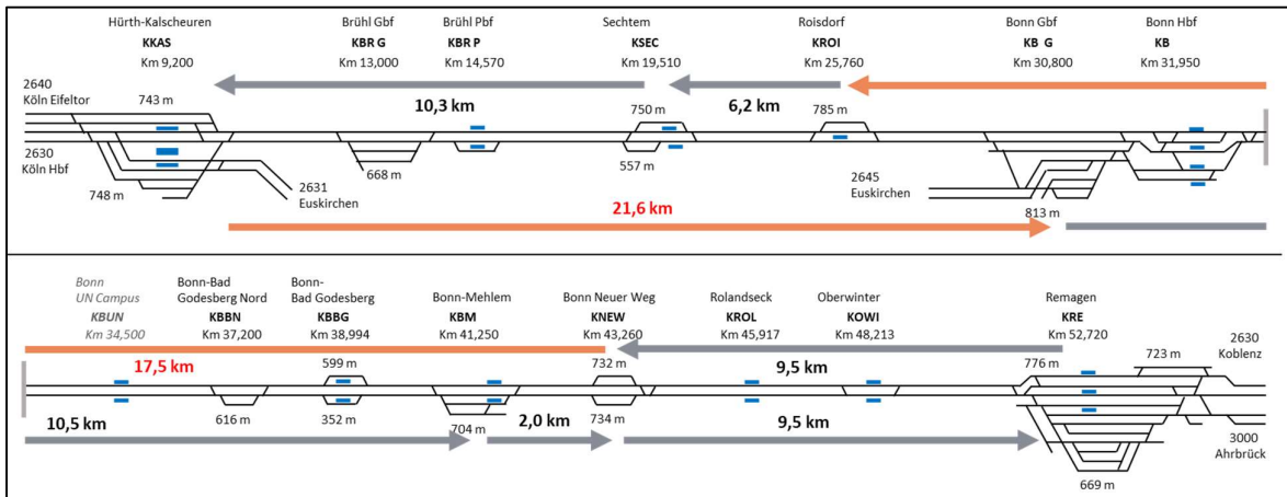
Abbildung 7: Abstände seitenrichtiger Überholungsgleise für 700 m lange Züge
