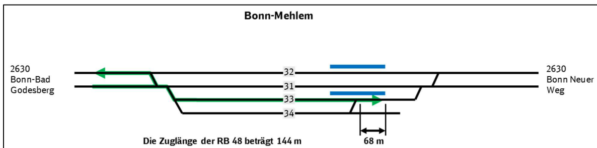
Abbildung 12: Schematischer Gleisplan des Bahnhofs Bonn-Mehlem
