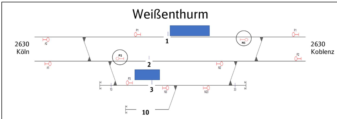
Abbildung 25: Zusätzliche Ausfahrtsignale N1 und P2 in Weißenthurm
