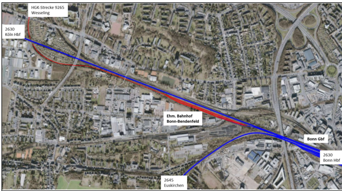
Abbildung 19: Anschluss an die HGK-Infrastruktur in Bonn-Bendenfeld
