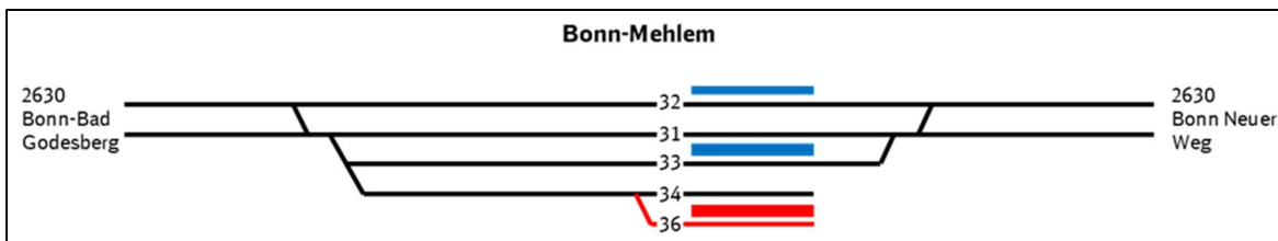
Abbildung 20: Spurplan Bonn-Mehlem nach Anpassung
