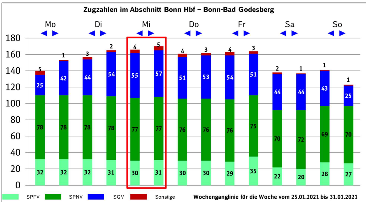
Abbildung 3: Wochenganglinie 25.01. - 31.01.2021 im Abschnitt Bonn Hbf - Bonn-Bad Godesberg
