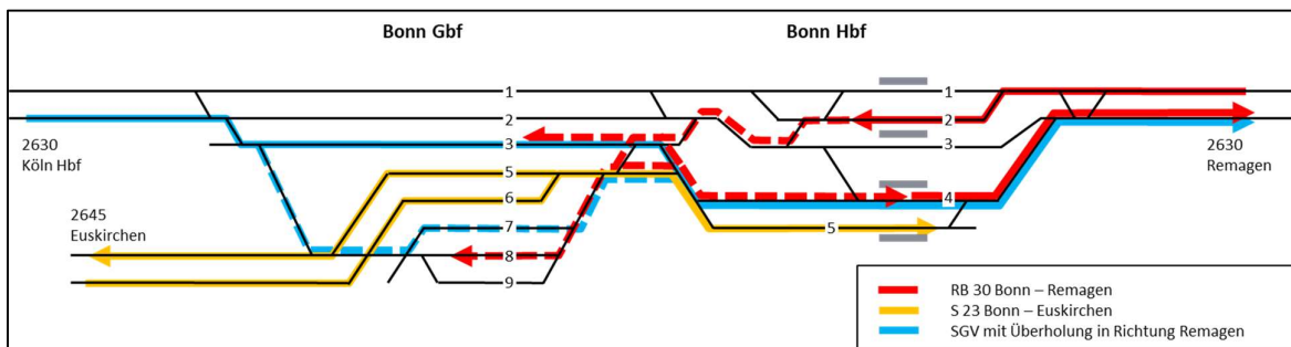
Abbildung 10: Fahrwegüberschneidungen im Bereich Bonn Hbf / Bonn Gbf
