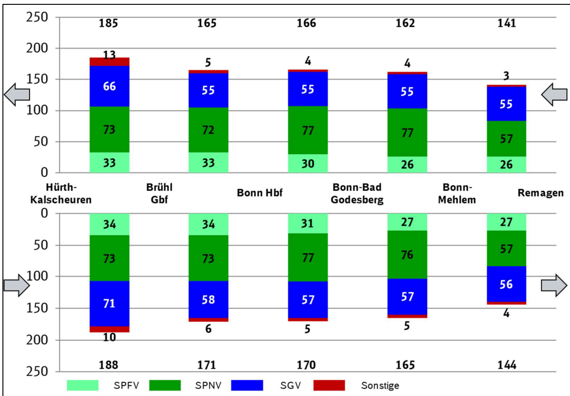
Abbildung 2: Abschnittsbezogene Zugzahlen nach Verkehrsarten
