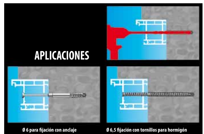
Bloques de hormigón
