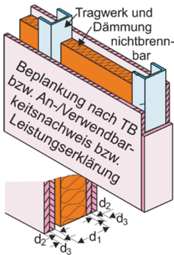
Abb. 3-2: Trockenbauweise mit nichtbrennbarem Tragwerk (Ständern)
