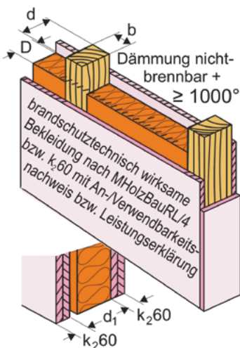
Abb. 3-3: Holzrahmen- und Holztafelbauweise nach MHolzbauRL Abschnitt 4
