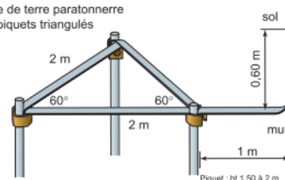
Prise de terre paratonnerre Système patte d'oie
