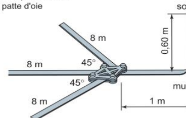
Prise de terre paratonnerre Système patte d'oie améliorée
