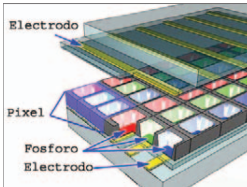
Otra imagen de la tecnología de plasma en la que se recoge un conjunto de celdas. Cada píxel esta compuesto por tres celdas coloreadas con cada uno de los colores primarios.
