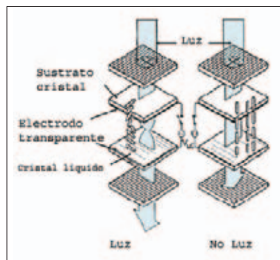
En este gráfico podemos ver de manera esquemática cómo funciona cada celda en la tecnología LCD y cómo se logra desviar, o no, la luz polarizada mediante impulsos eléctricos.
