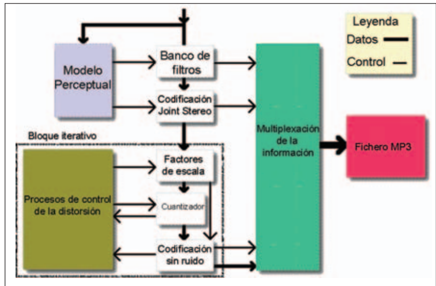
El diagrama de bloques de MP3 muestra la cantidad de tareas implicadas en la compresión, que aún es mayor en los nuevos algoritmos para otros formatos.
