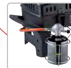
Optional für den mobilen Einsatz: Kartuschenhalter-Set (Art.-Nr. 2092) und Schraubkartusche (Art.-Nr. 6322)
