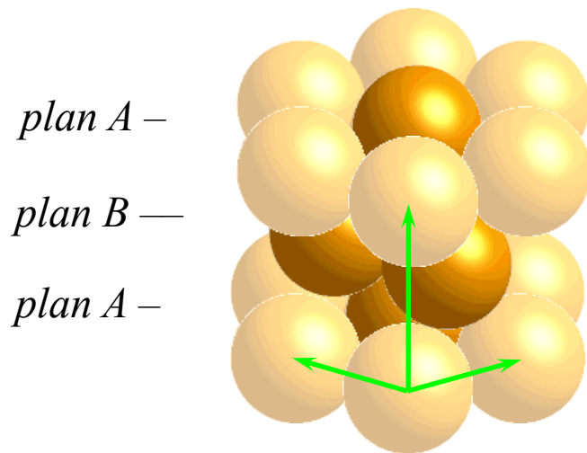
Maille hexagonale
