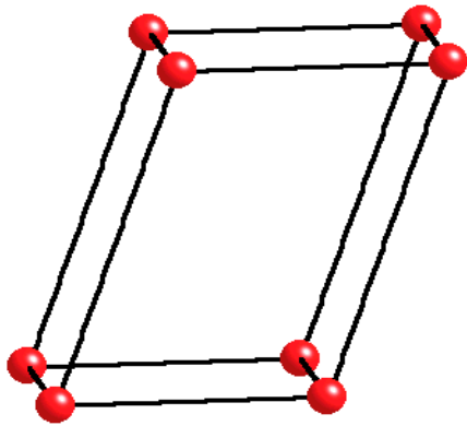
triclinique P
