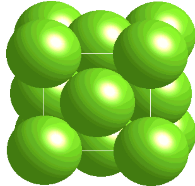
Cubique F : 74 %
