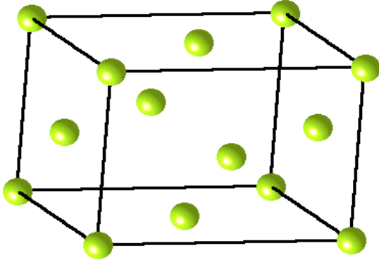
Orthorhombique F
