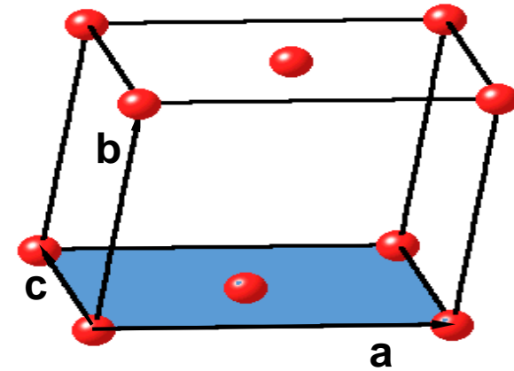
monoclinique B
