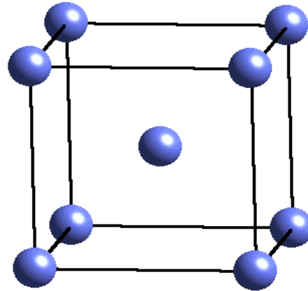
Cubique I
