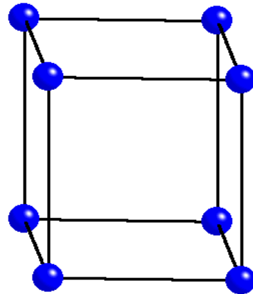
monoclinique P
