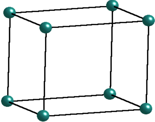
Orthorhombique P
