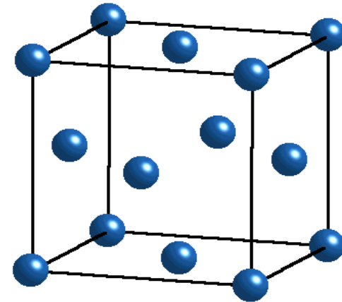
Cubique F
