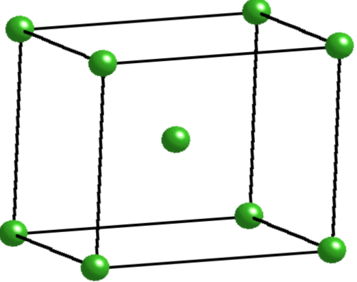
Orthorhombique I
