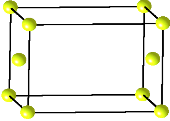
Orthorhombique A
