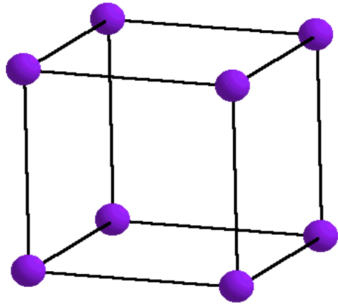
Cubique P
