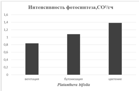
Рисунок 1 – Интенсивность фотосинтеза в тканях листьев Platanthera bifolia
