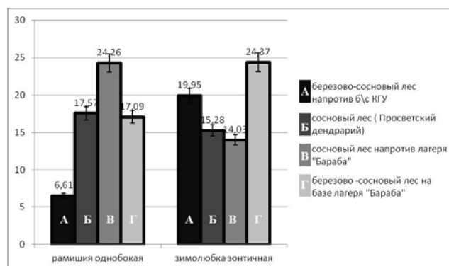
Рисунок 1 – Содержание хлорофилла в листьях Chimaphila umbellata и Ortilia secunda
