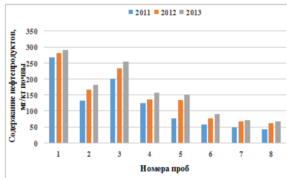
Рисунок 1 – Содержание нефтепродуктов в почве анализируемых проб
