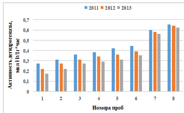
Рисунок 3 – Результаты определения активности дегидрогеназы почвы
