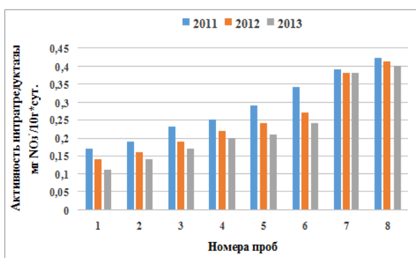
Рисунок 5 – Изменение активности нитратредуктазы почвы
