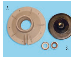
A. Models P4RA, P4EA, P6RA & P6EA
